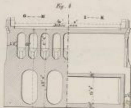
Querschnitte
