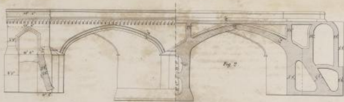
AUFRISS
