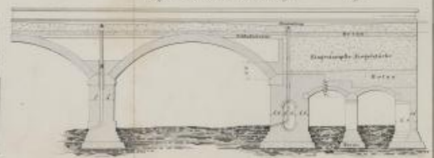
Längsschnitt der Endauflage Fig. 4
