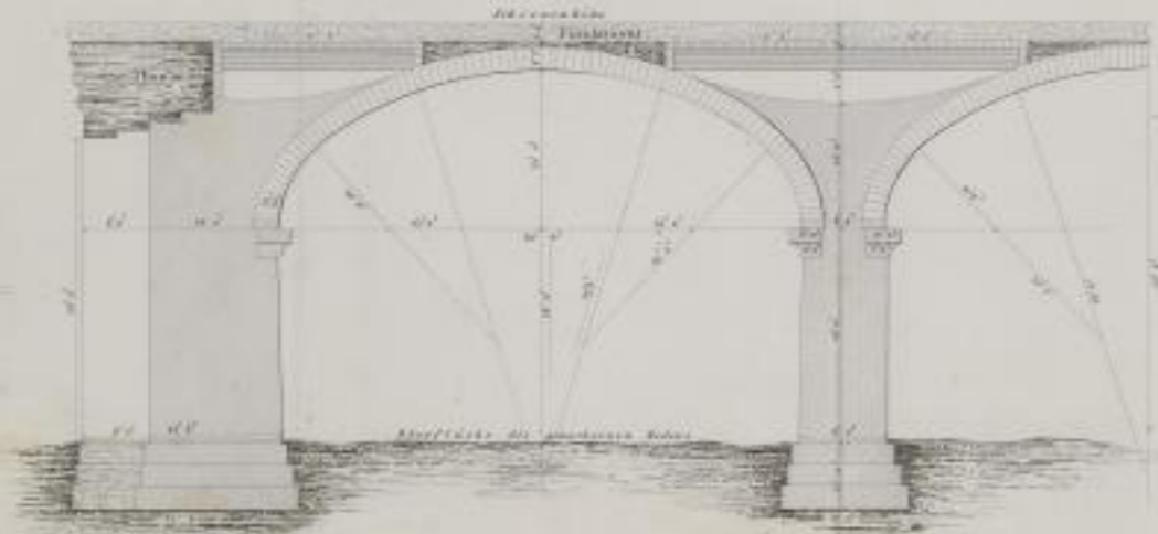
Fig. 4 LONGUE SECTION DEUX DES ARCHES
