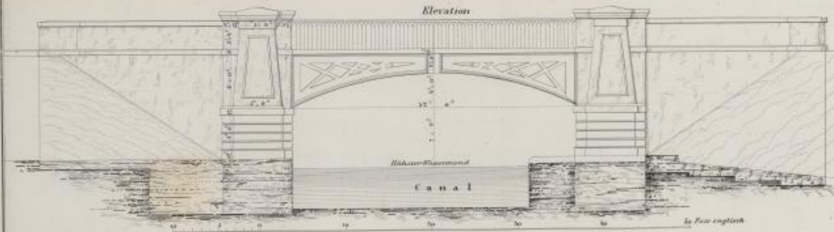
Elevation
