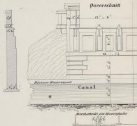
Querschnitt
