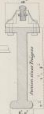
Figur zur Verbindung zw. den Mauerplatten
