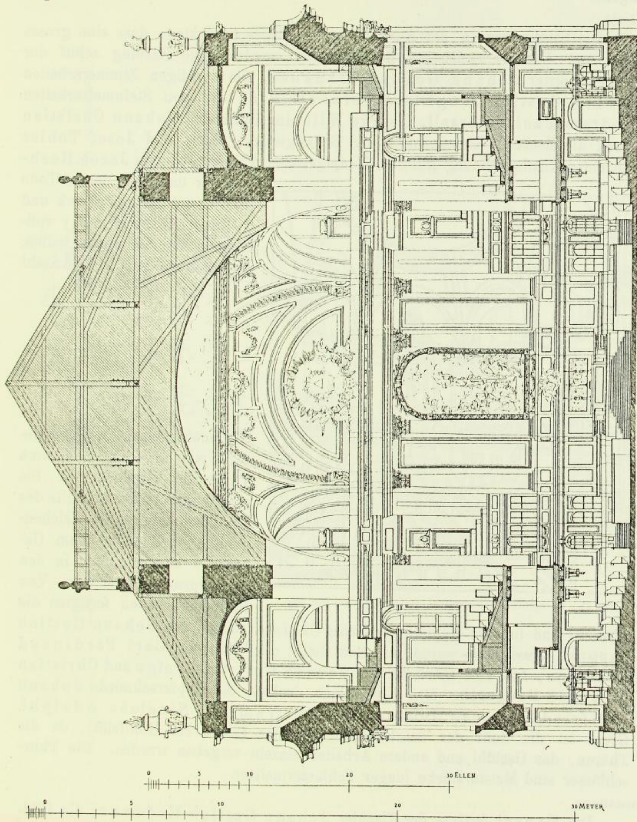
Fig. 20. Querschnitt durch die Kreuzkirche, nach der Originalzeichnung Hölzers.
