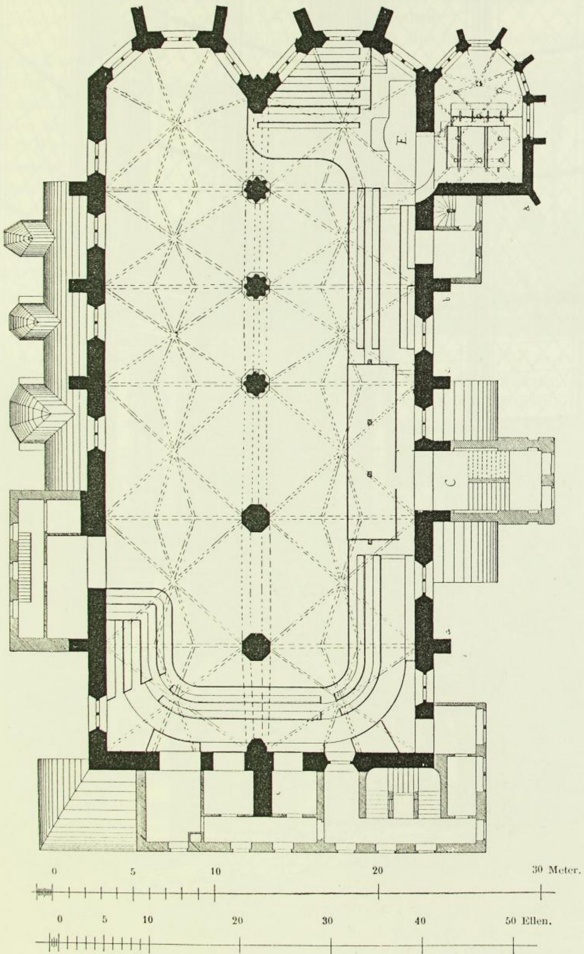
Fig. 50. Franziskanerkirche, Grundriss des Emporengeschosses. Zustand vor 1864. C. Thurm von 1736. E. Orgel von 1720. 6*
