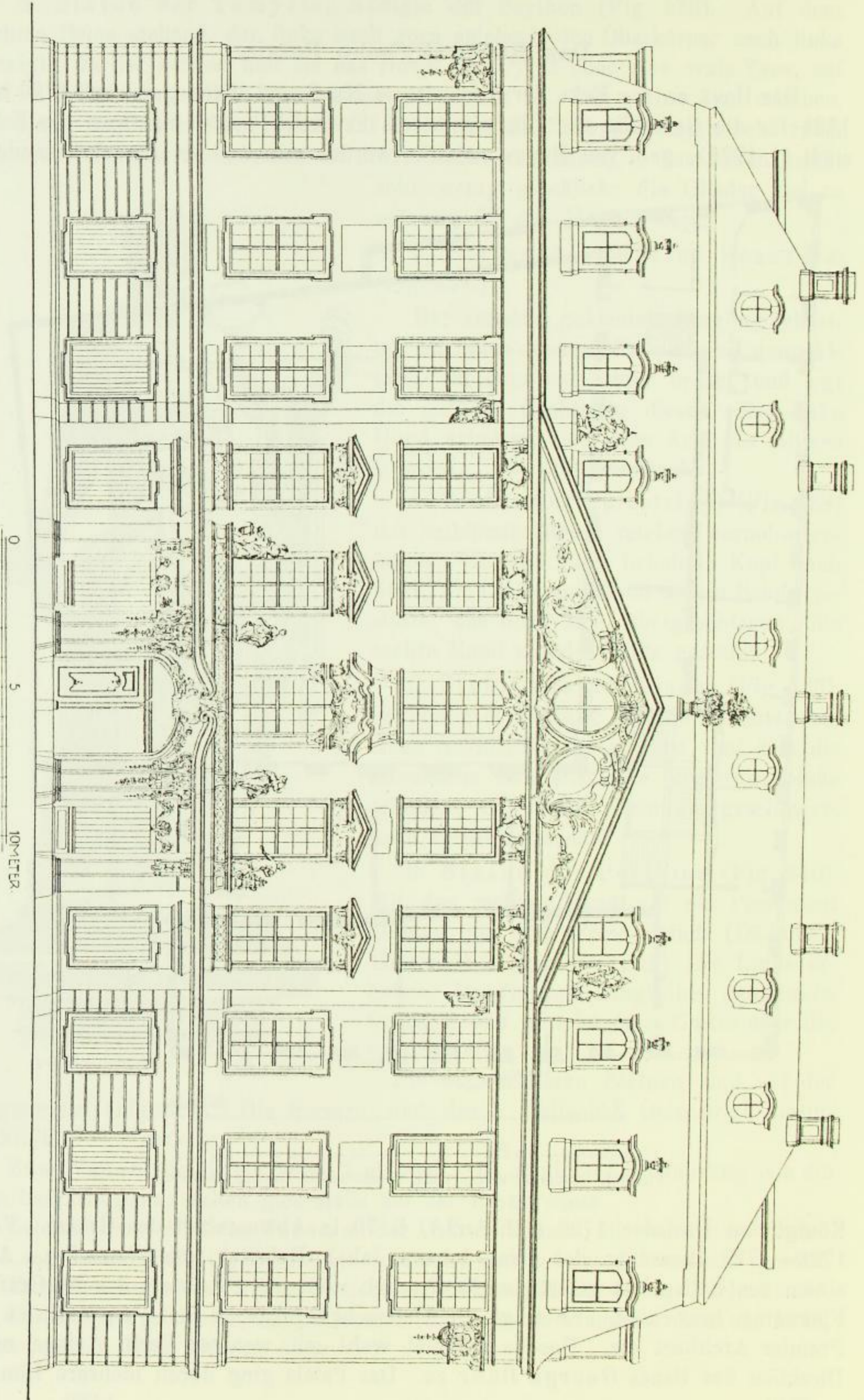
Fig. 442. Rutowsky'sches Palais. Ansicht gegen die Kreuzstrasse.
