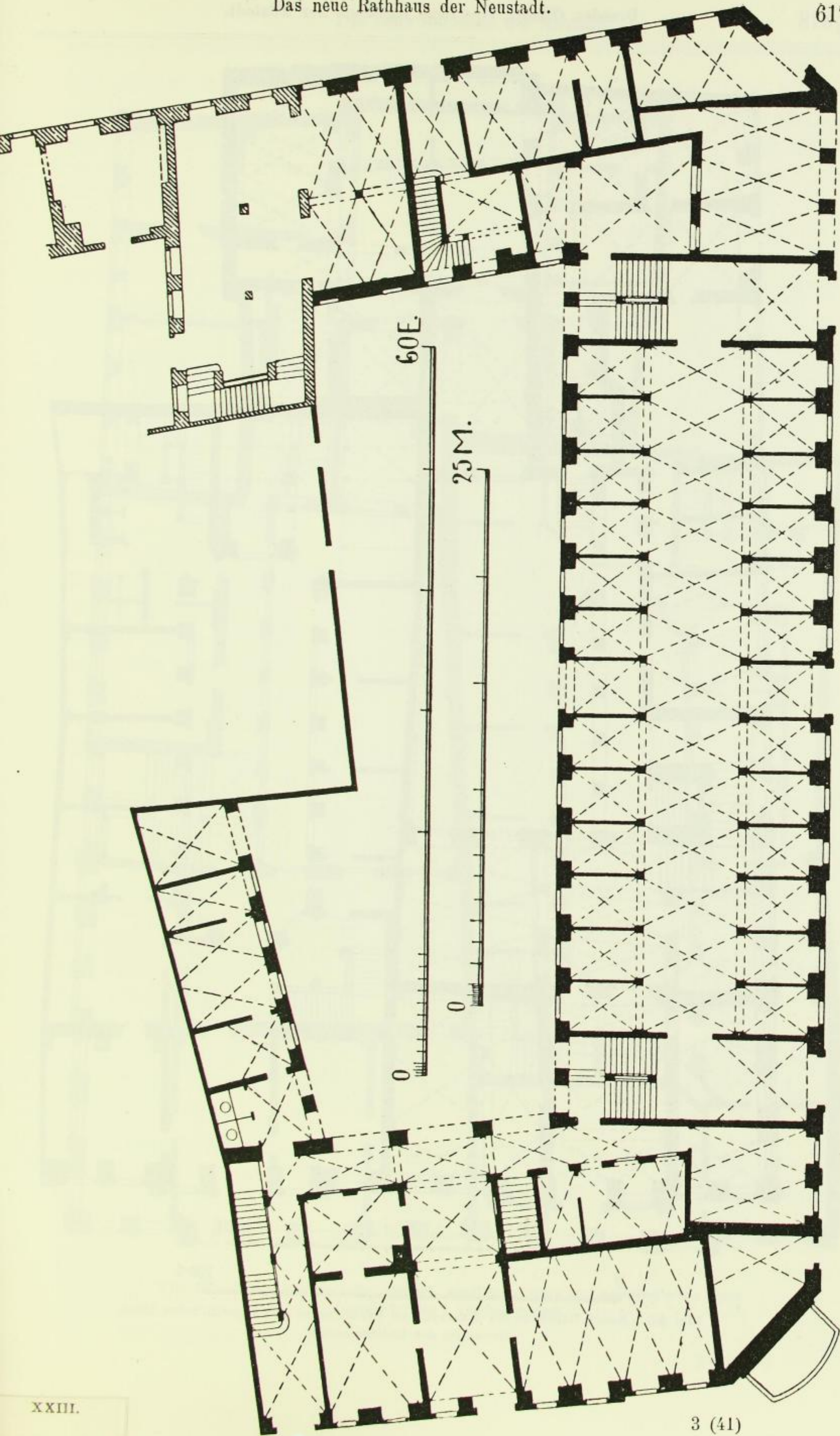
Fig. 464. Neues Rathhaus der Neustadt. Grundriss des Erdgeschosses.
