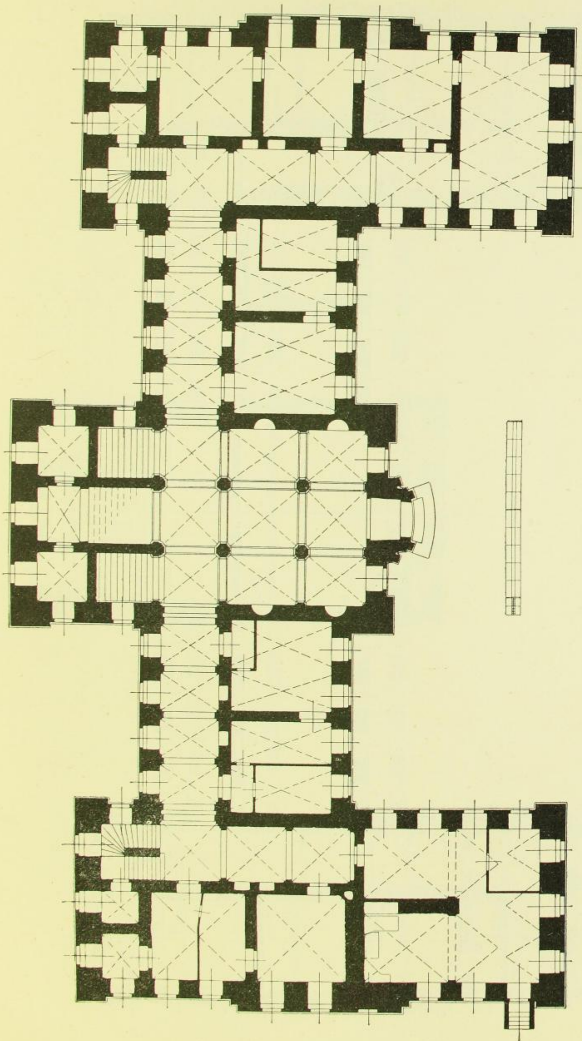
Fig. 57. Joachimstein, Schloß, Grundriß des Erdgeschosses.
