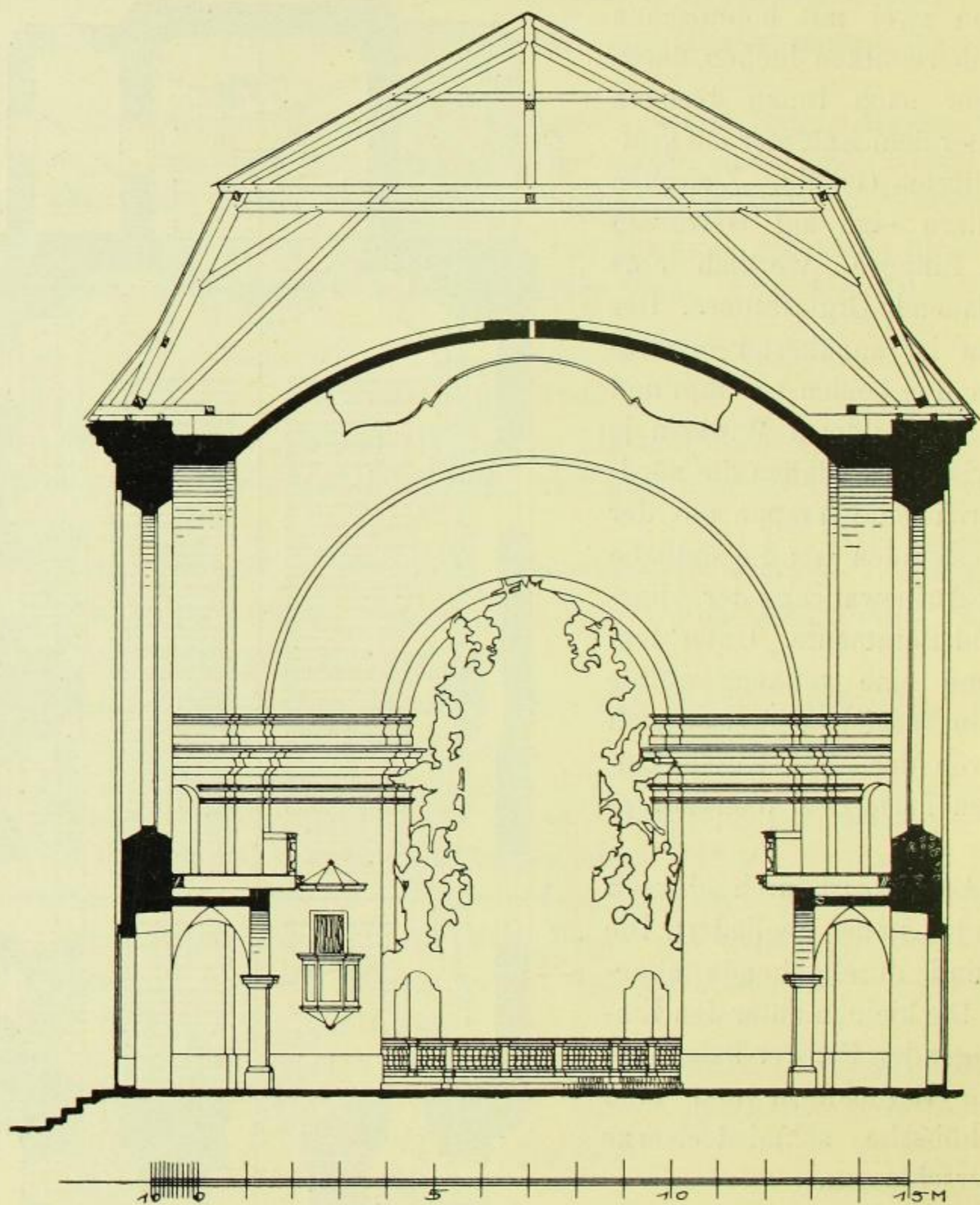
Fig. 85. Königshain, katholische Kirche, Querschnitt.
