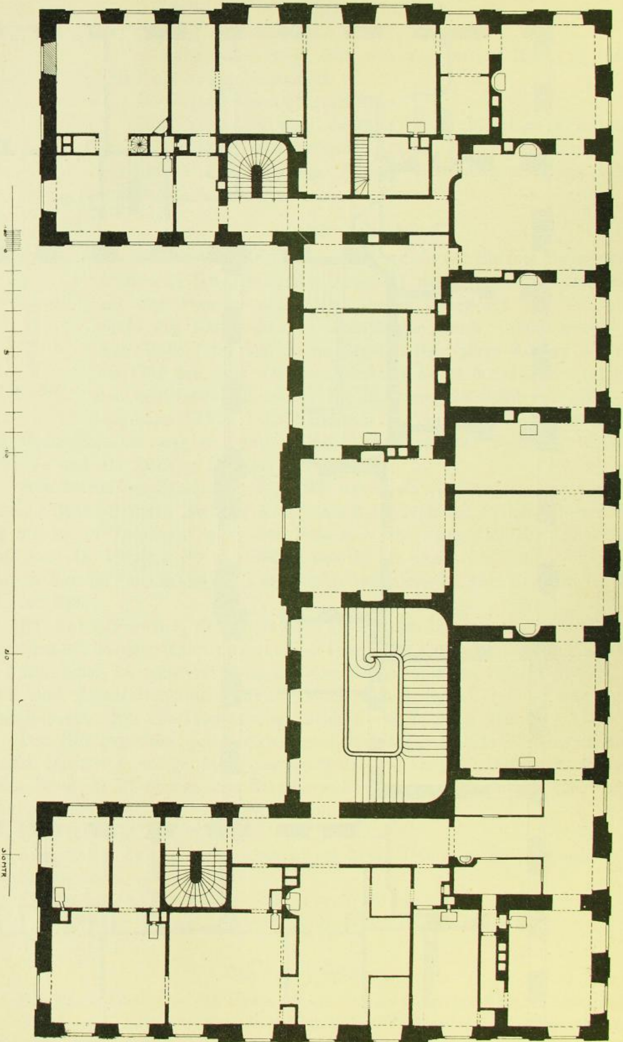
Fig. 207. Reibersdorf, Schloß, Grundriß des Obergeschosses.
