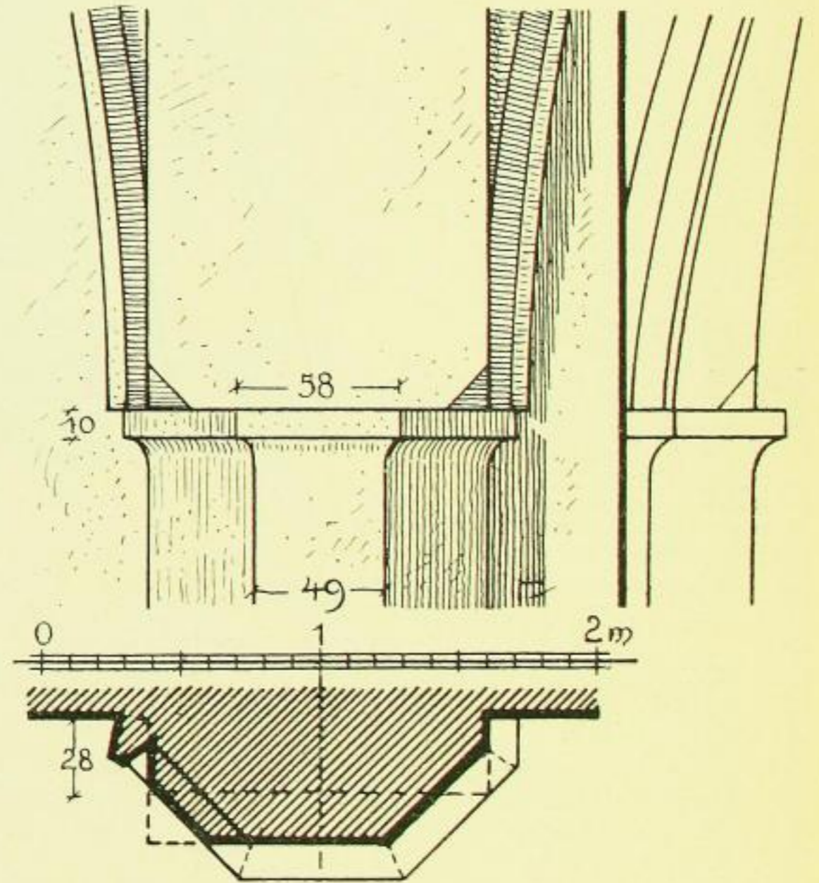
Fig. 145. Marienstern, Klosterkirche, Profil der Pfeilersockel.
