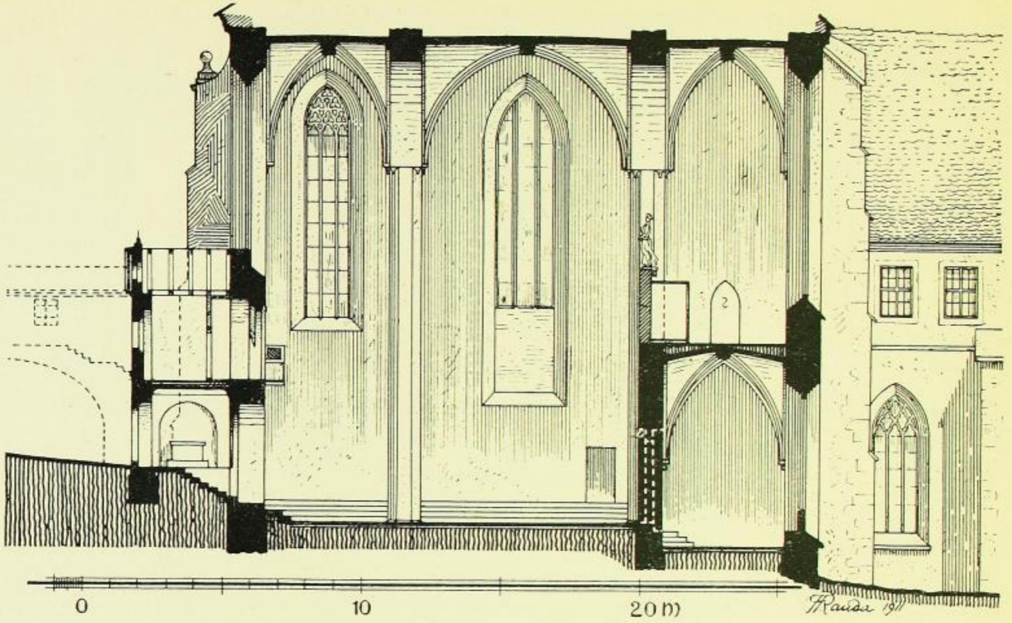
Fig. 144. Marienstern, Klosterkirche, Querschnitt.
