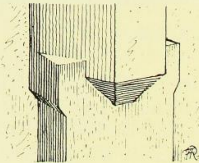
Fig. 147. Marienstern, Klosterkirche, Wandpfeiler auf der Ostseite.
