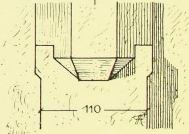
Fig. 148. Marienstern, Klosterkirche, Wandpfeiler auf der Ostseite mit Gewölbe-Anfänger.
