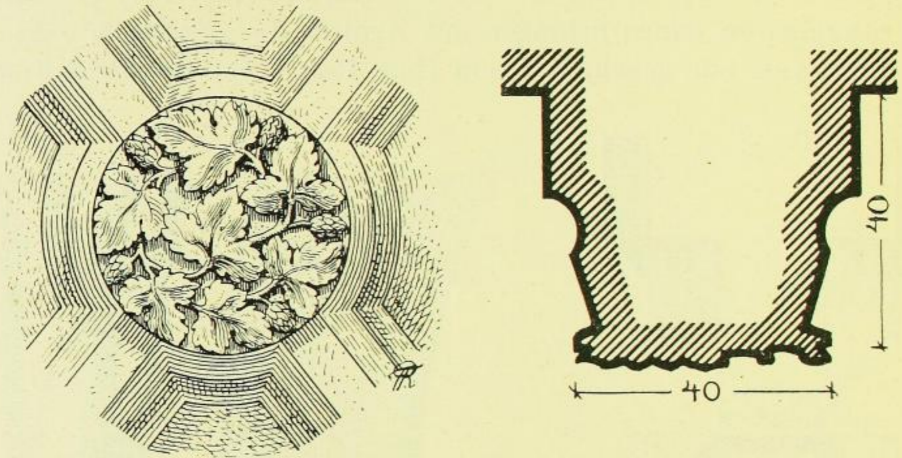
Fig. 154 u. 155. Marienstern, Klosterkirche, Schlußstein, Unteransicht und Querschnitt.
