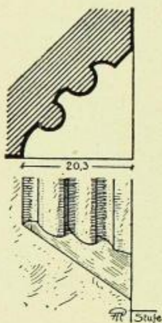
Fig. 159. Marienstein, Klosterkirche, Profil des Westtors.
