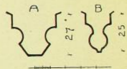
Fig. 163. Marienstein, Klosterkirche, Rippenprofile des Gewölbes unterm Nonnenchor.
