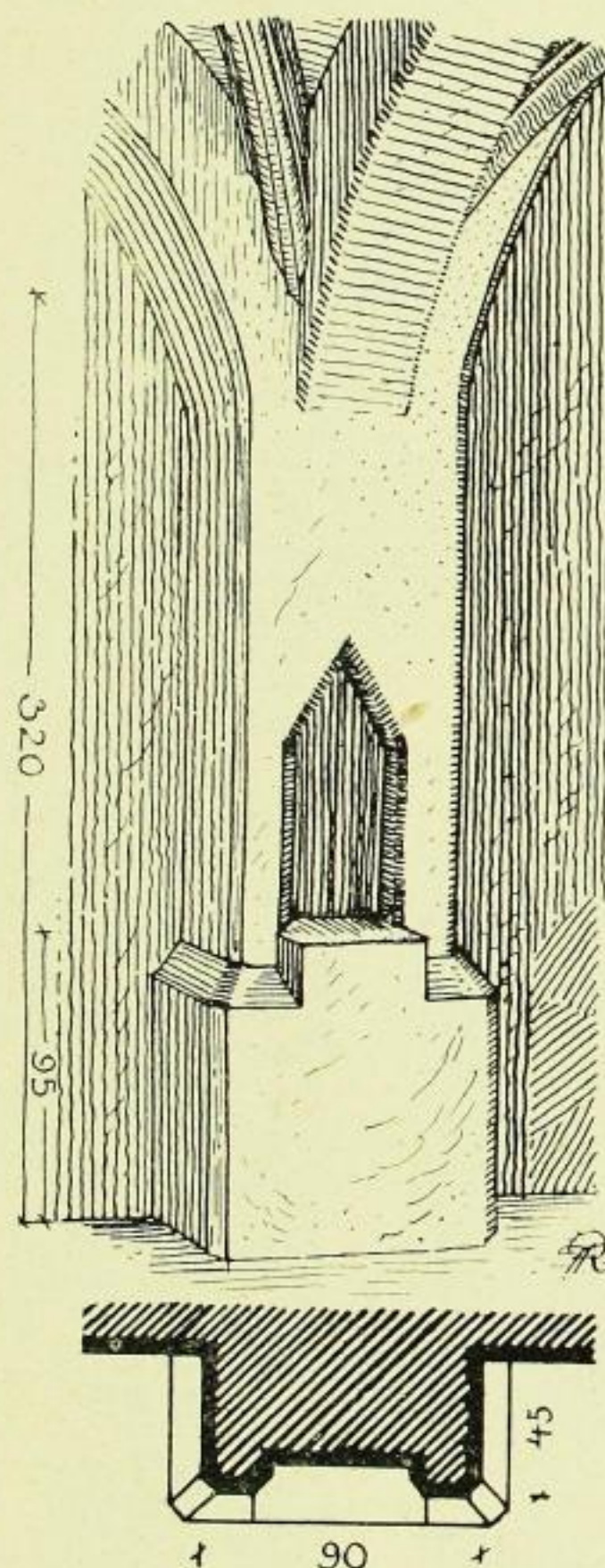
Fig. 192. Marienstern, Kloster, Ostpfeiler im Kapitelsaal.
