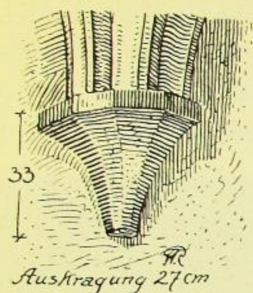
Fig. 185. Marienstern, Kloster, Gewölbekragstein in der Kreuzkapelle.
