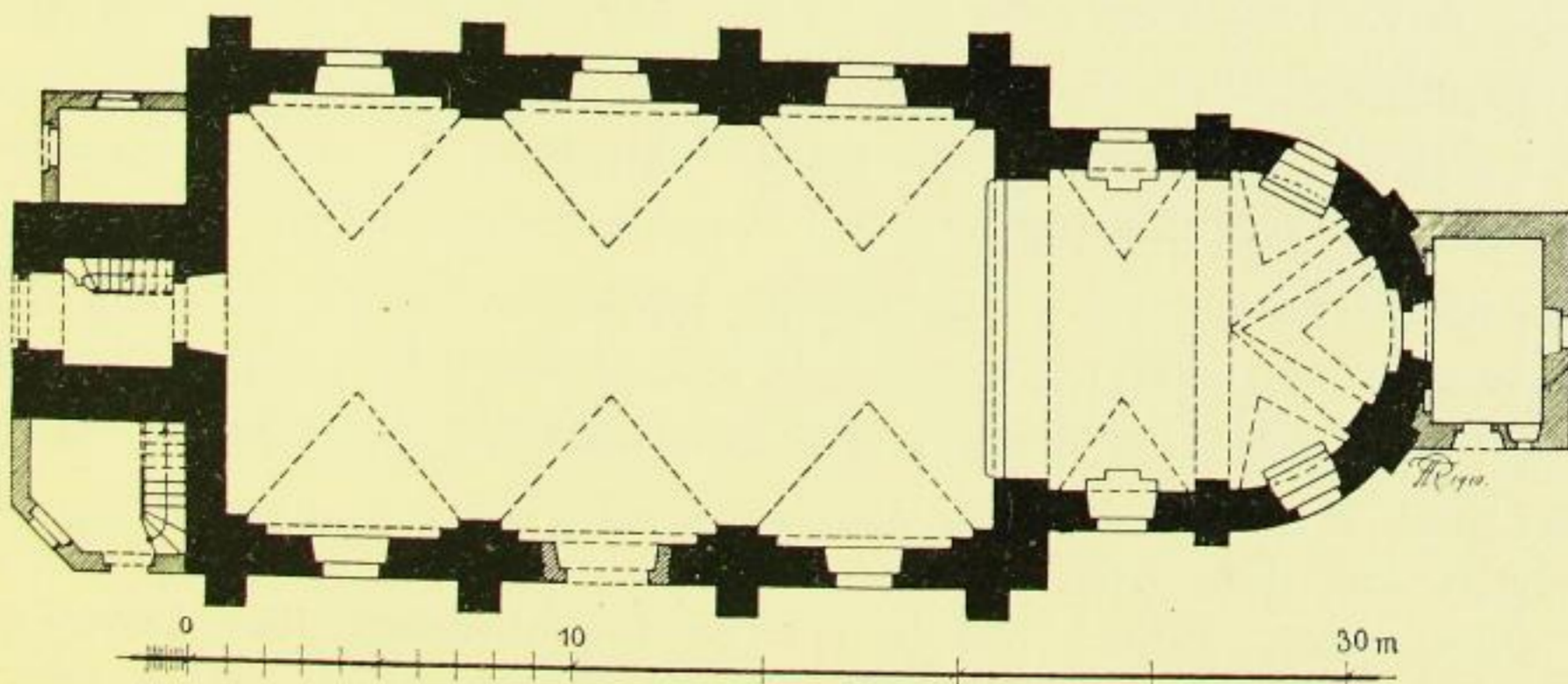
Fig. 306. Ralbitz, Kirche, Grundriß.
