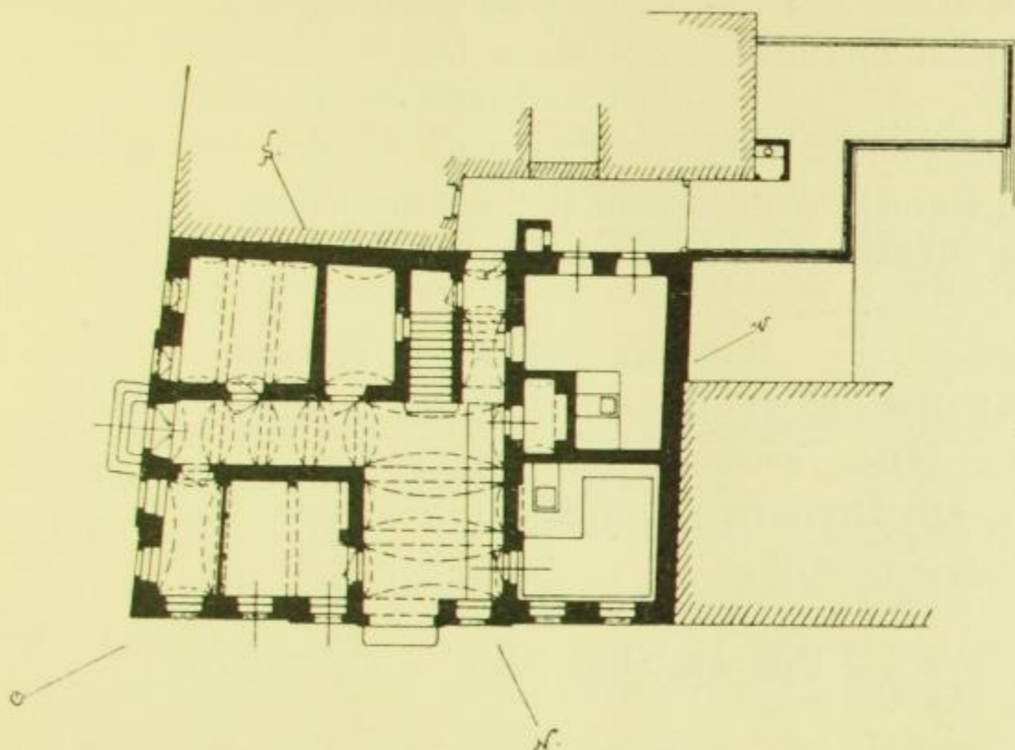
Fig. 27. Bernstadt, Neuere Rathaus, Erdgeschoß.
