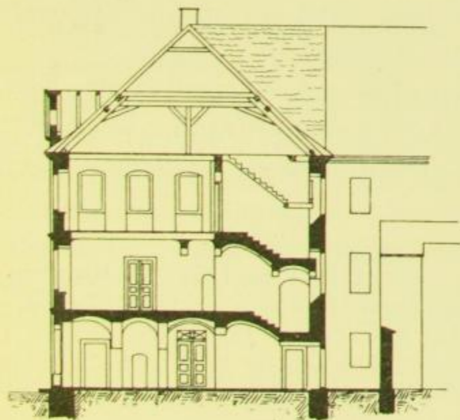
Fig. 30. Bernstadt, Neuere Rathaus, Querschnitt.
