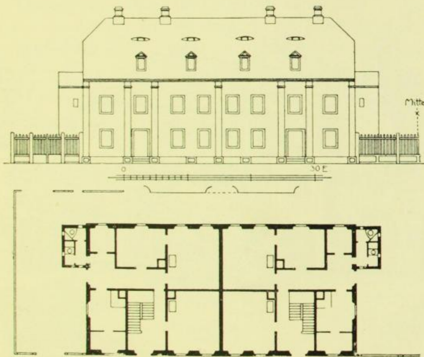
Fig. 45 und 46. Berthelsdorf, Unitätsdirektorenhäuser, Schauseite und Grundriß.
