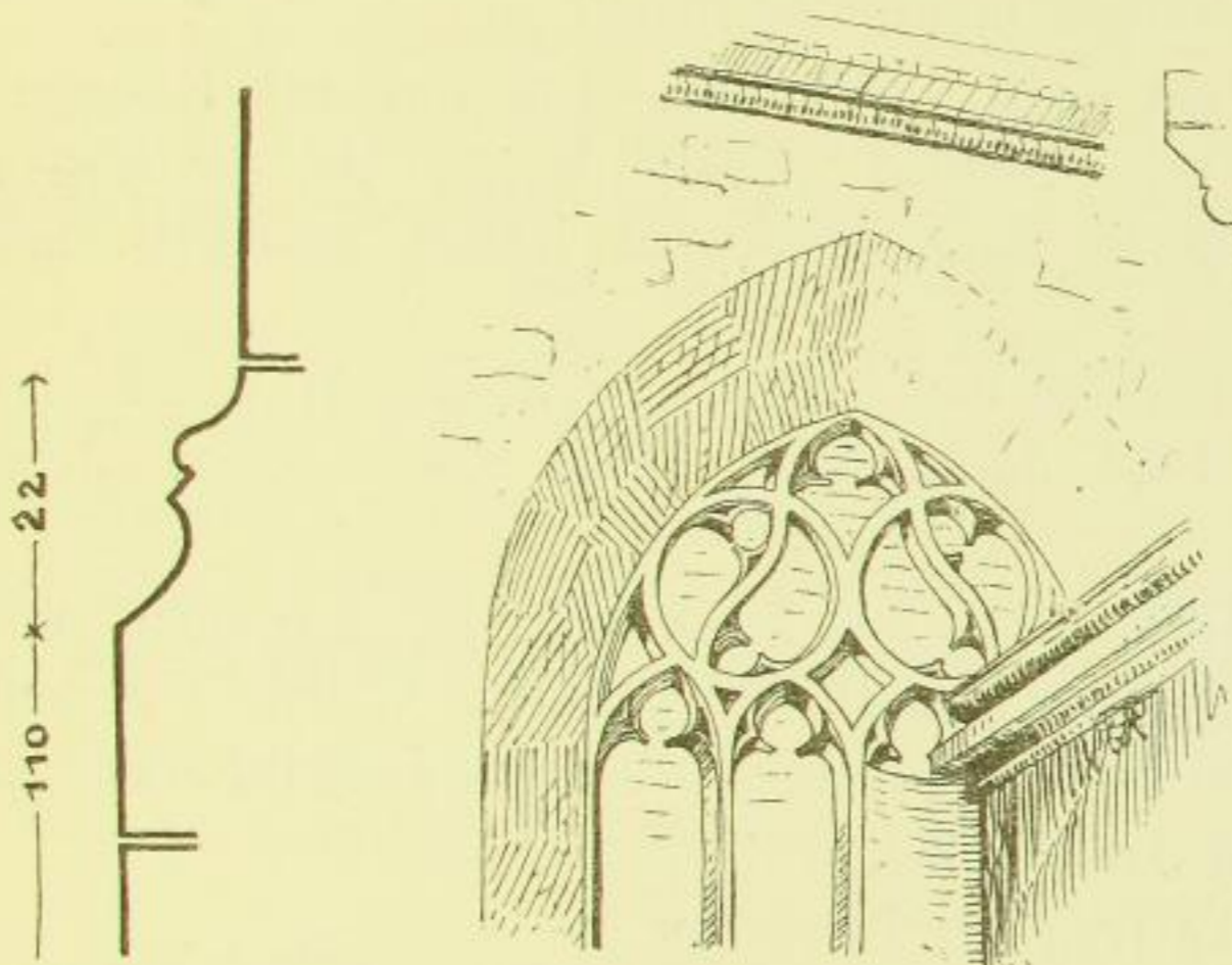
Fig. 72. Michaeliskirche, Sockelprofil.
