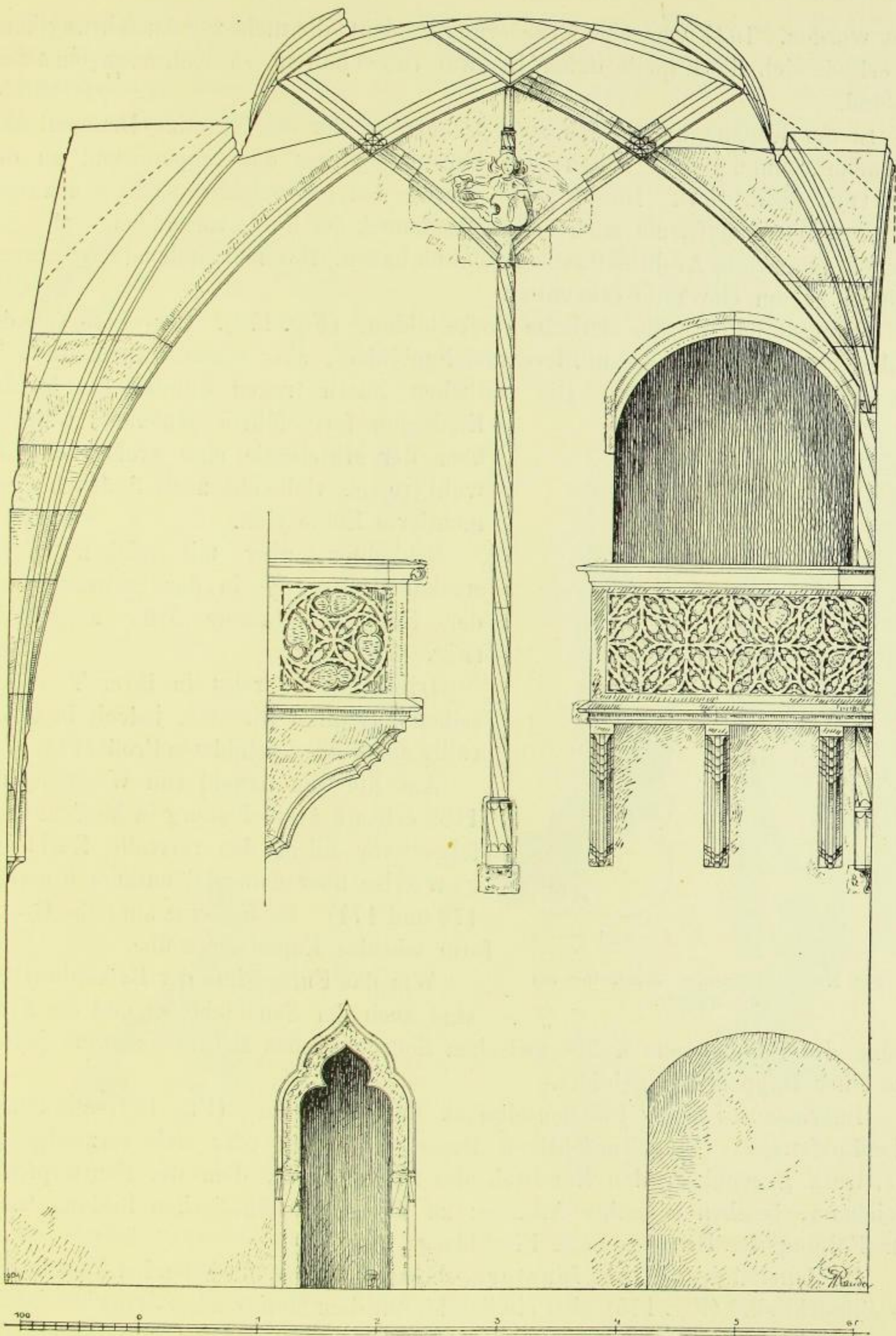
Fig. 169. Schloßkapelle, Schnitt (mit ergänztem Gewölbe).
