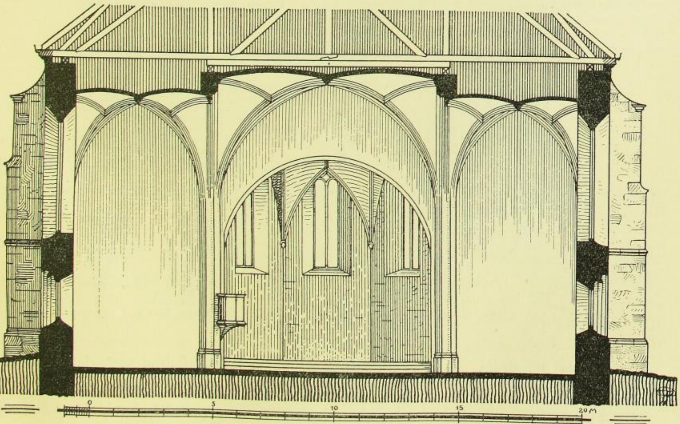
Fig. 49. Göda, Kirche, Querschnitt durch das Langhaus.
