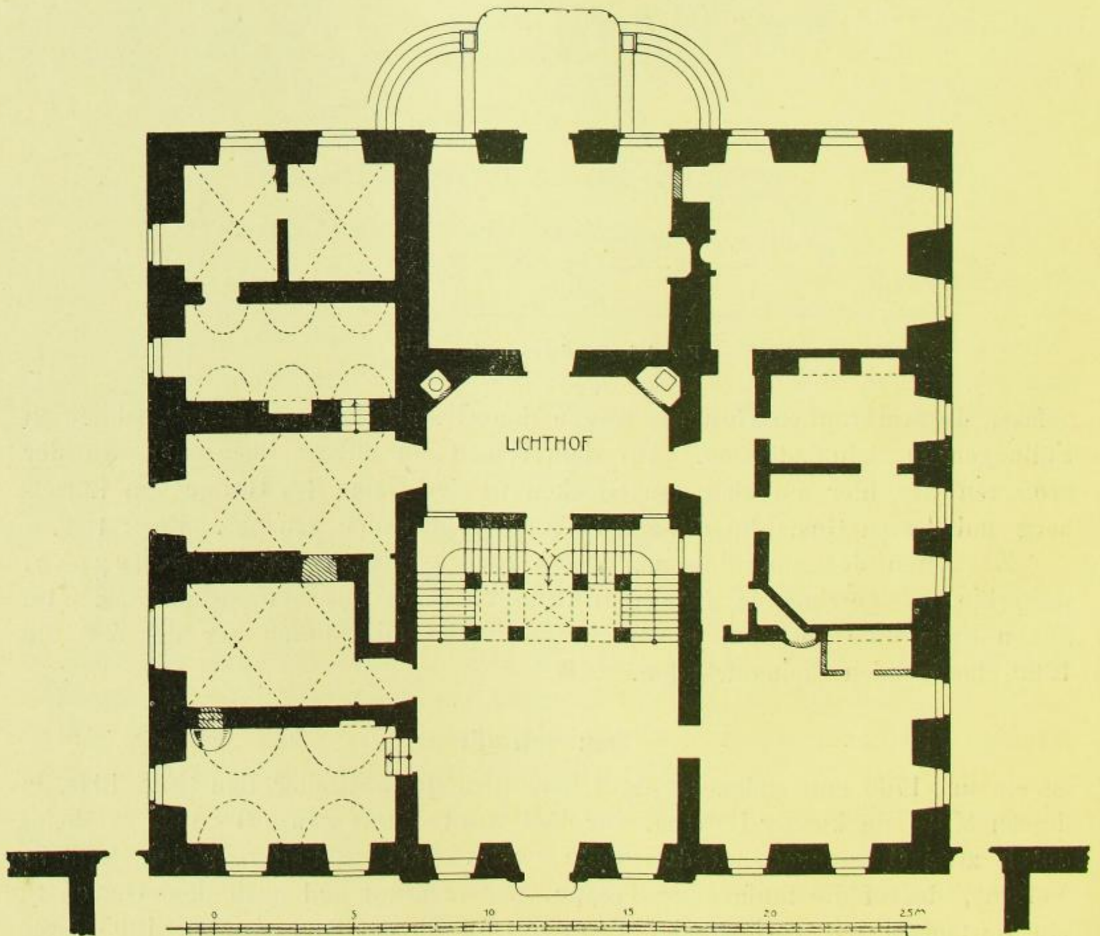
Fig. 197. Niedergurig, Schloß, Erdgeschoß.
