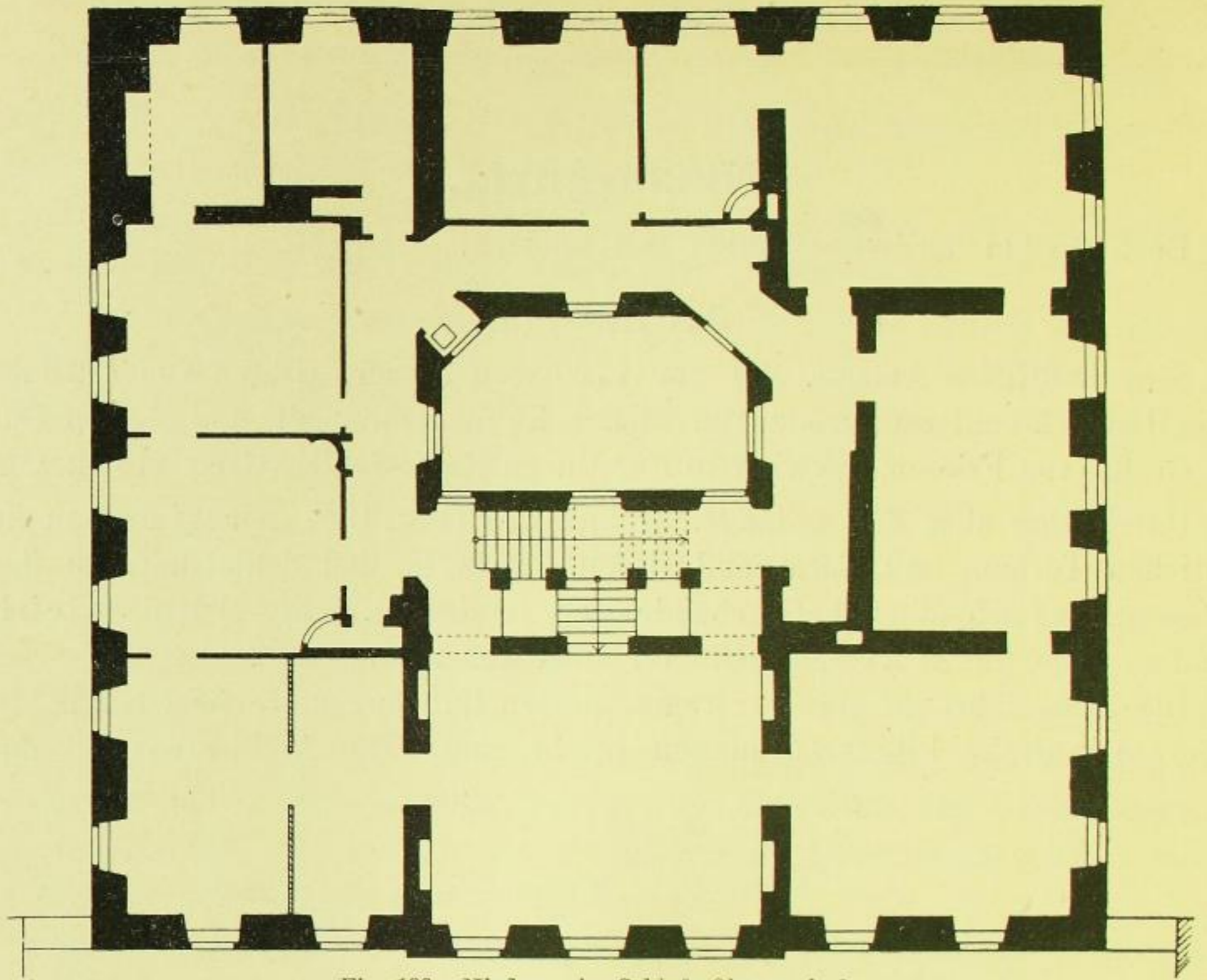
Fig. 196. Niedergurig, Schloß, Obergeschoß.
