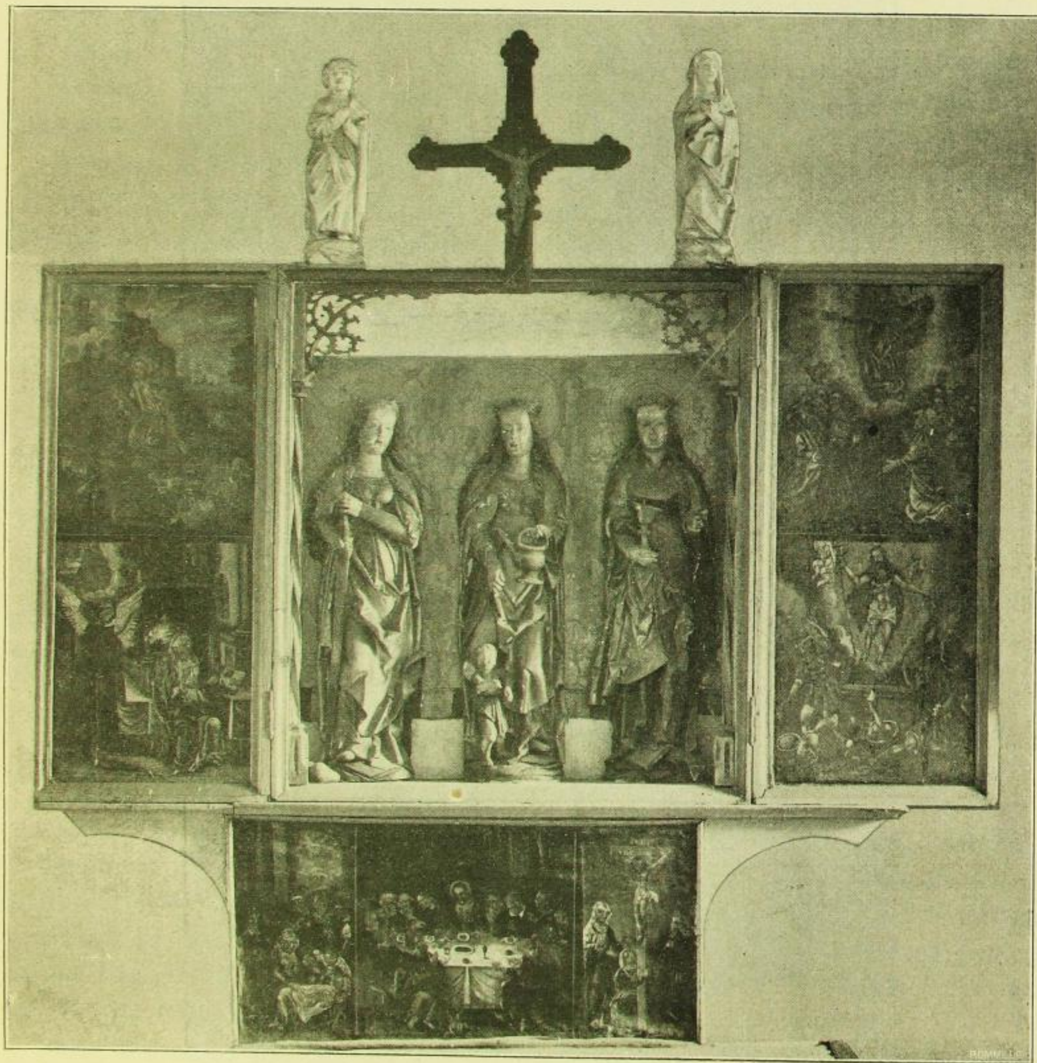
Fig. 38. Börtewitz, Altarschrein.
