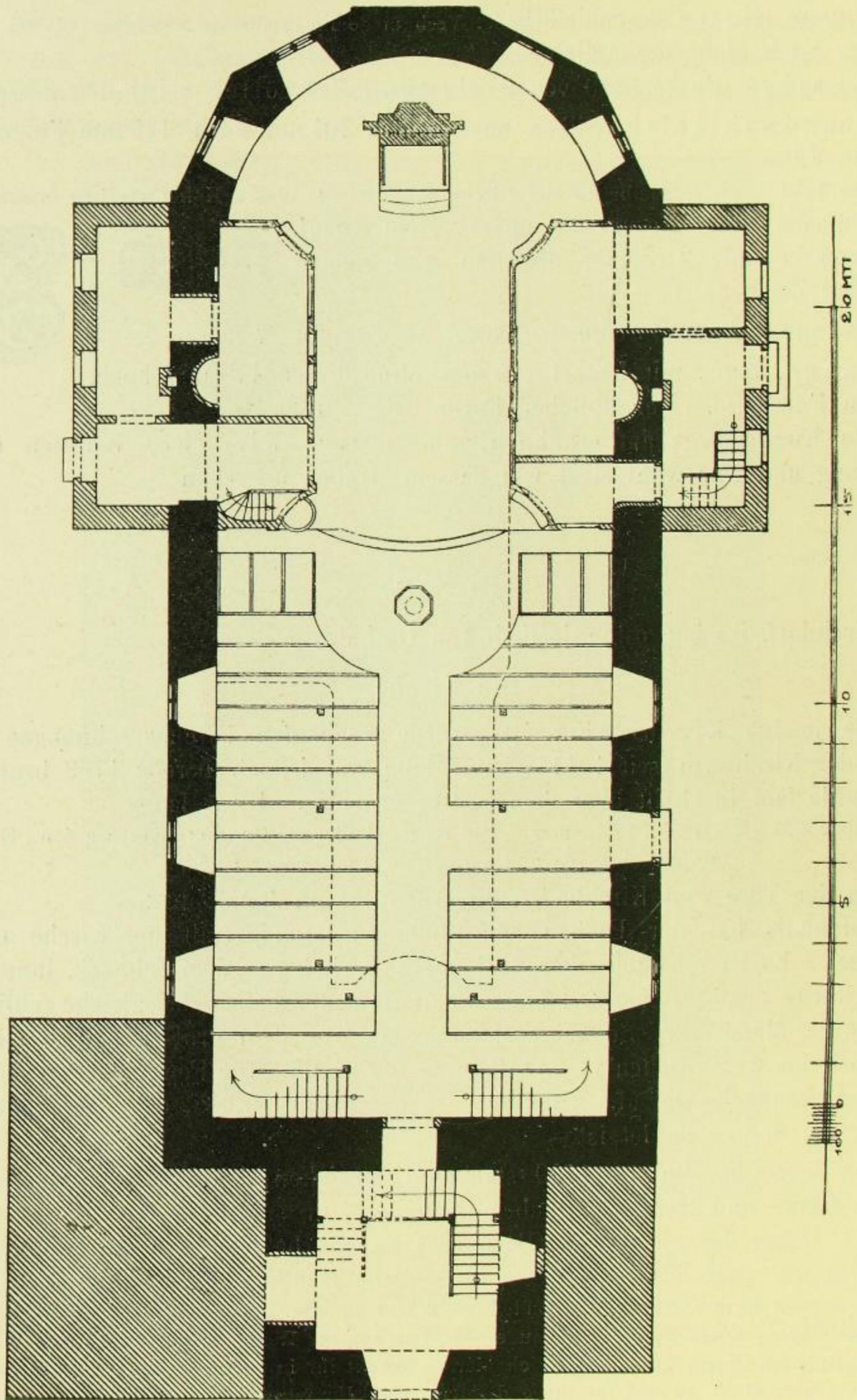
Fig. 40. Borna, Kirche, Grundriß.
