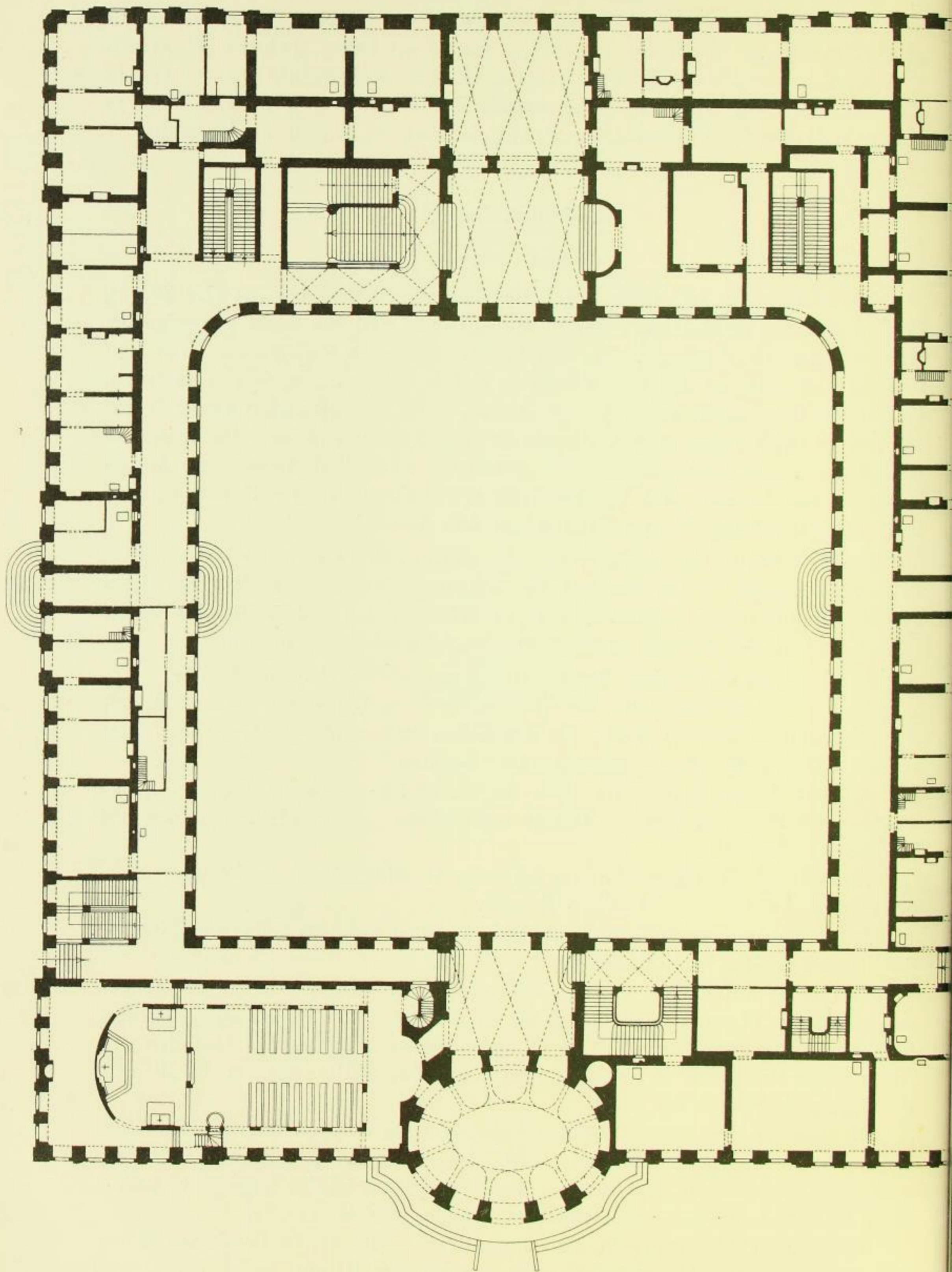
Fig. 132. Hubertusburg, Schloß, Grundriß des Erdgeschosses.
