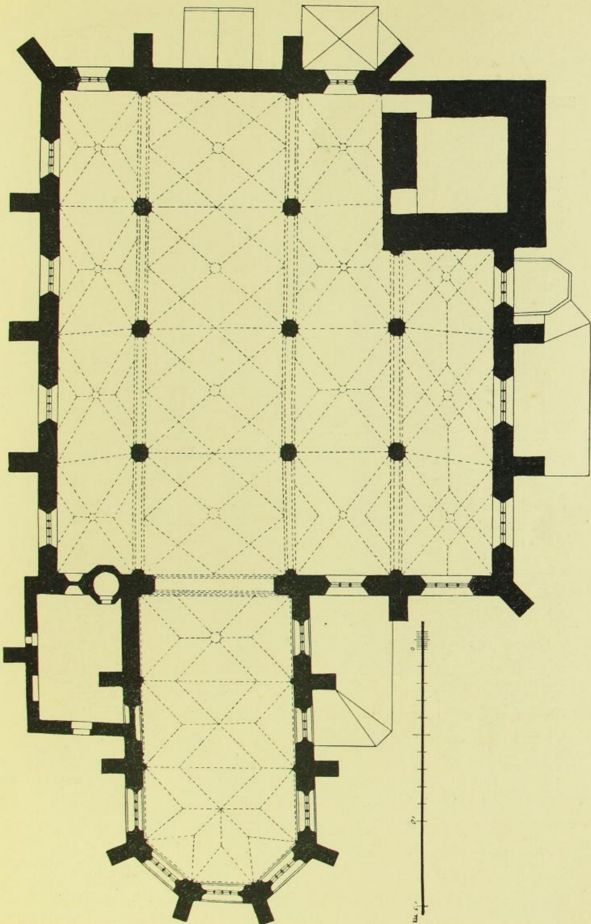
Fig. 4. Hauptkirche, Gewölbe-Grundriß.
