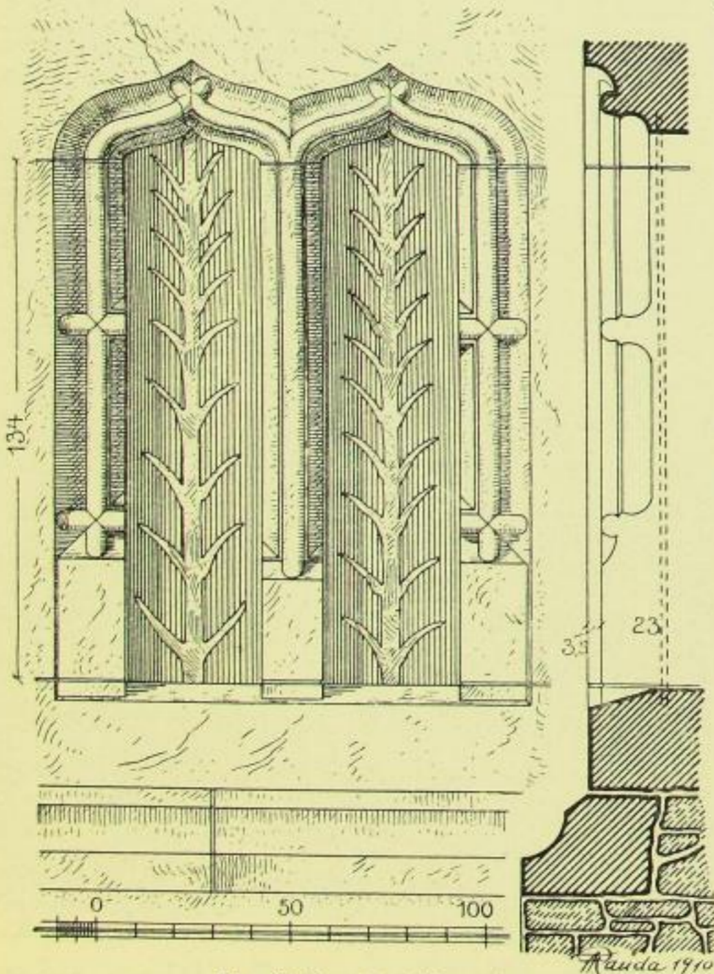
Fig. 306. Gruftfenster.
