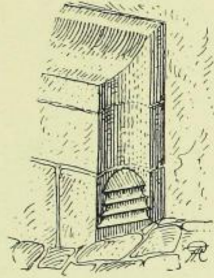
Fig. 309. Sockelgesims, Abschluß.
