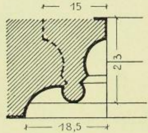
Fig. 313. Gewände vom Gruftfenster.
