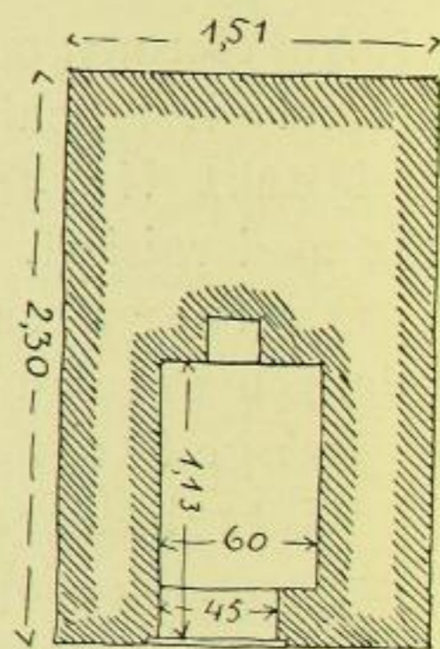
Fig. 357. Sepulchrum. Querschnitt und Grundriß, Hauptkirche.
