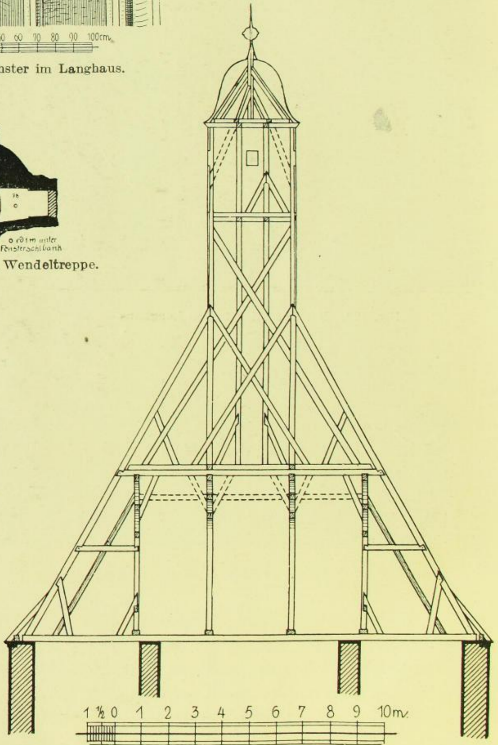
Fig. 134. Kirche, Dach, Schnitt.
