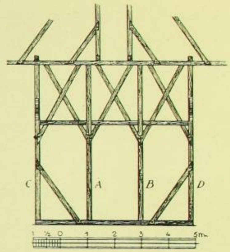
Fig. 135. Kirche, Dach, Seitenansicht.
