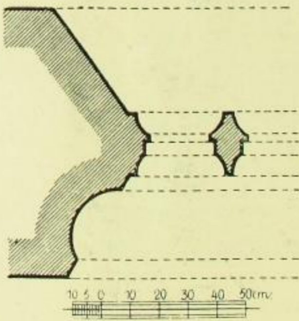
Fig. 138. Kirche, Chorfenster, Profil.
