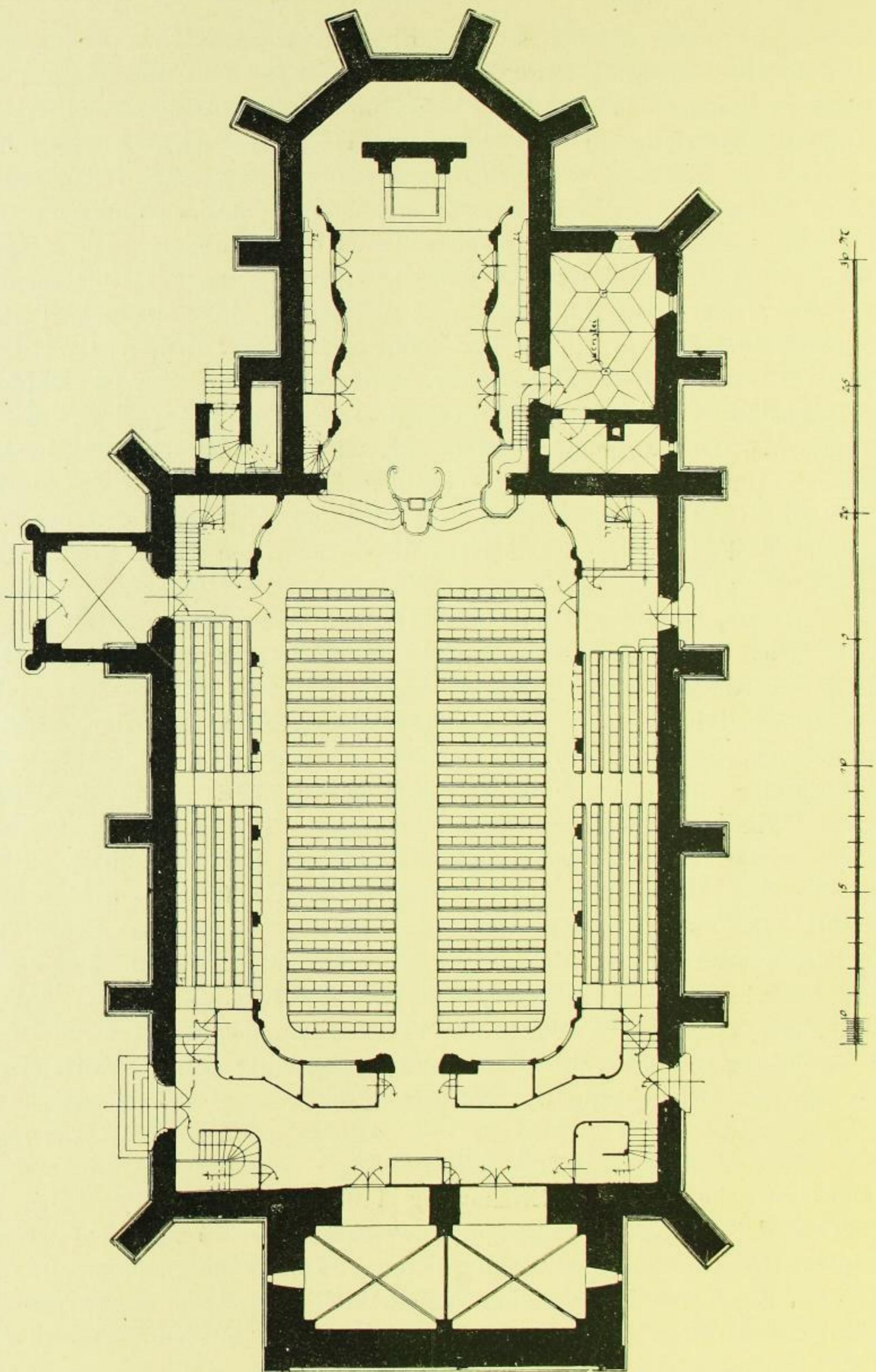
Fig. 359. Lommatzsch, Kirche, unterer Grundriß. Zustand vor 1900.
