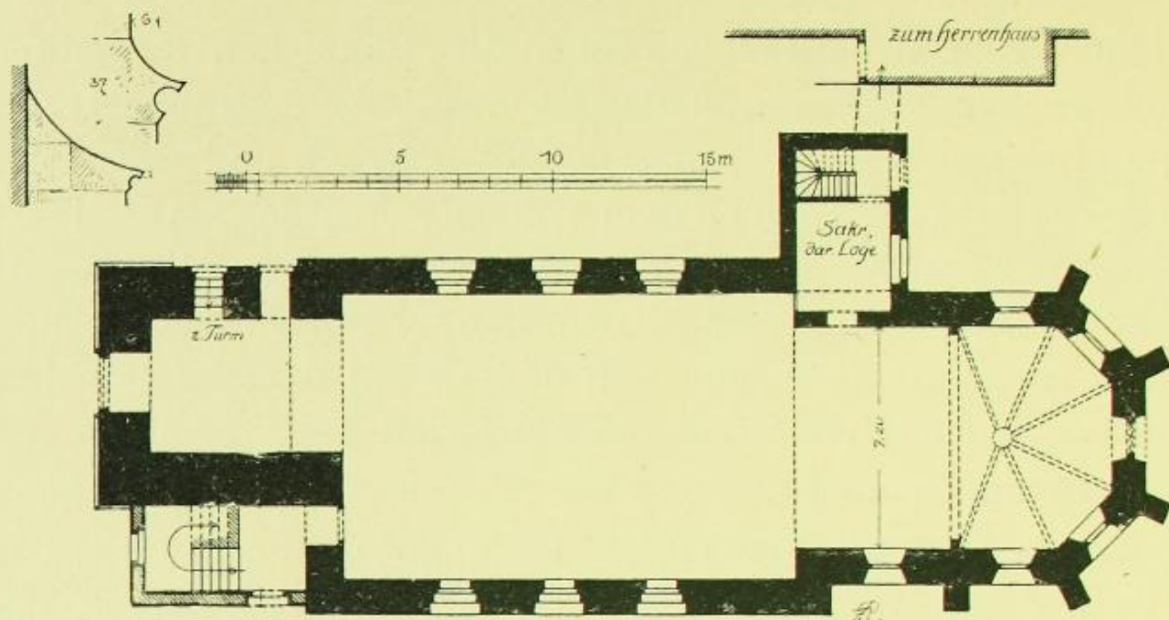
Fig. 620. Weistropp, Kirche, Grundriß.
