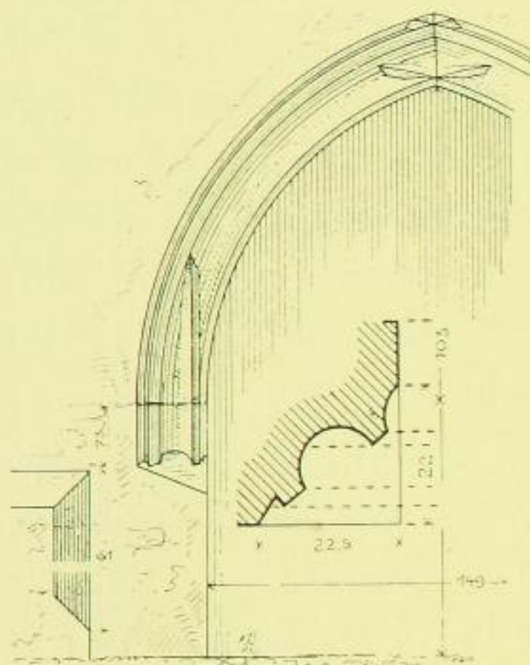
Fig. 621. Weistropp, Kirche, Tor.
