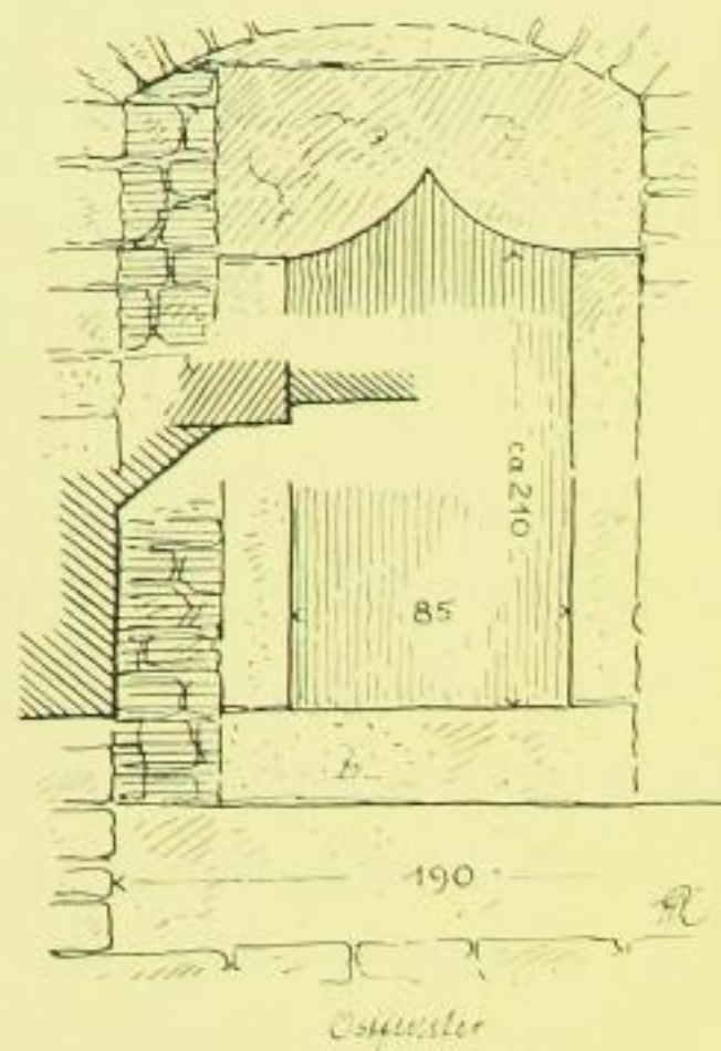
Fig. 623. Weistropp, Kirche, Turmfenster.
