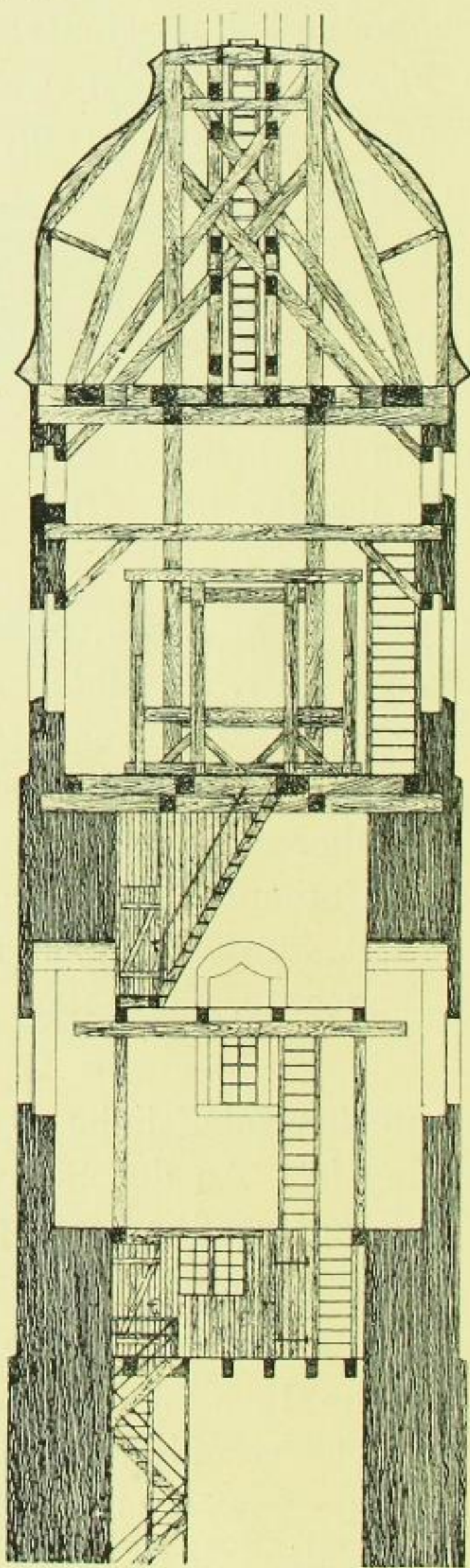
Fig. 622. Weistropp, Kirche, Dachreiter.
