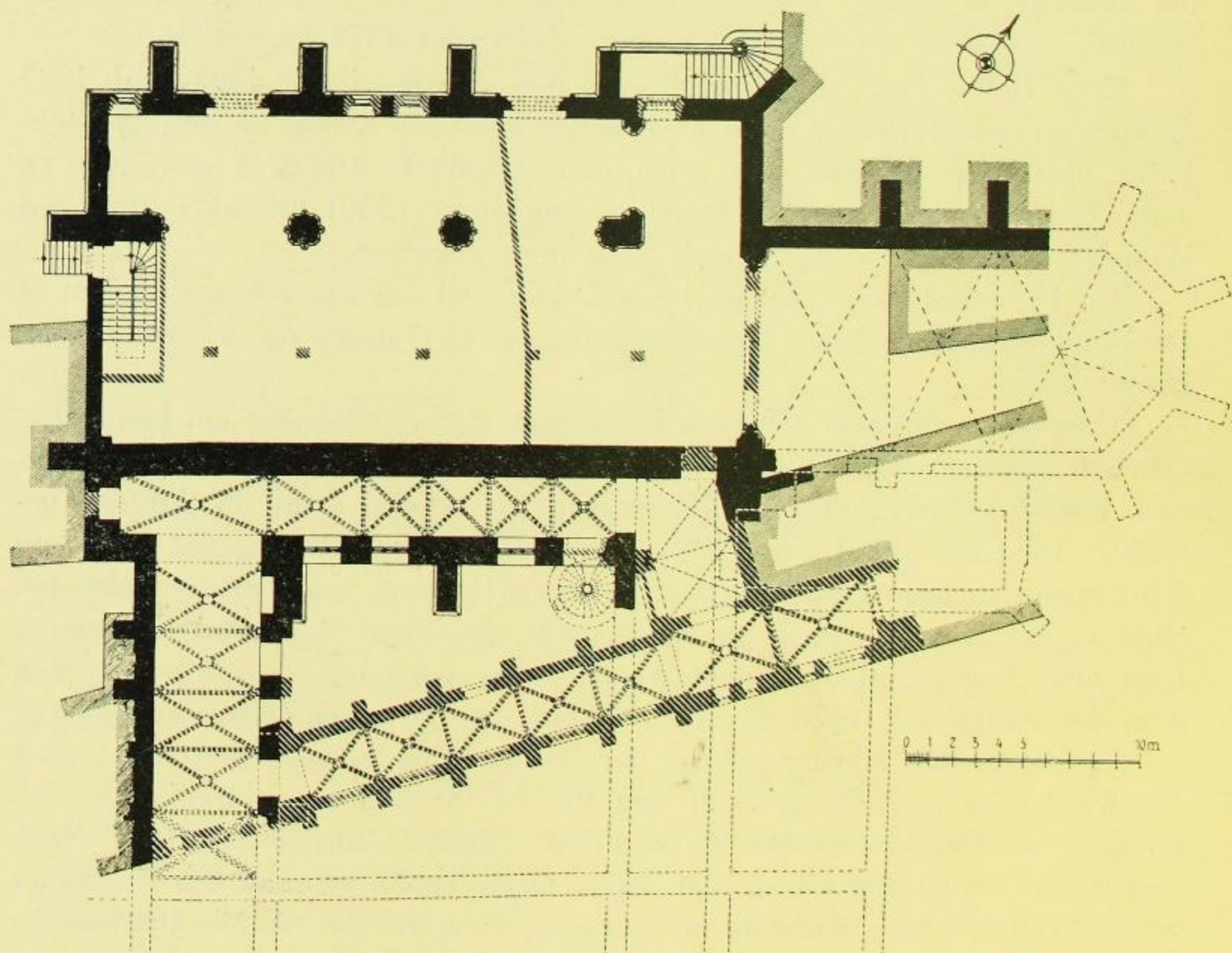
Fig. 92. Franziskanerkirche, Grundriß des Schiffes mit ergänztem Chor und Kreuzgang. Zustand nach 1900.
