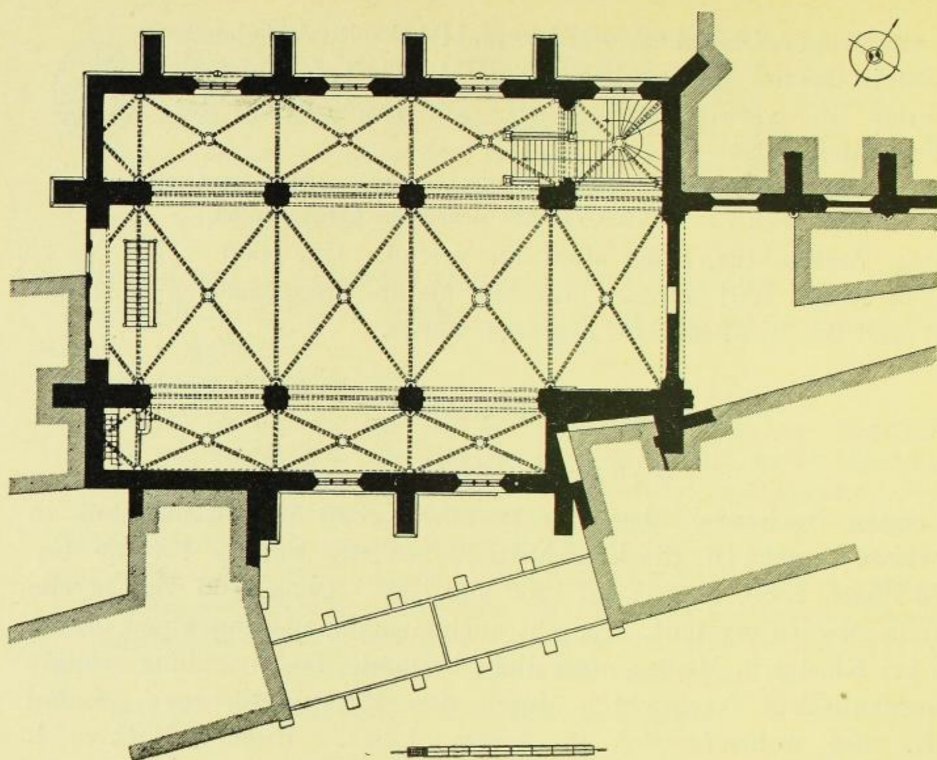
Fig. 91. Franziskanerkirche, Grundriß in Höhe des Obergeschosses. Zustand nach 1900.
