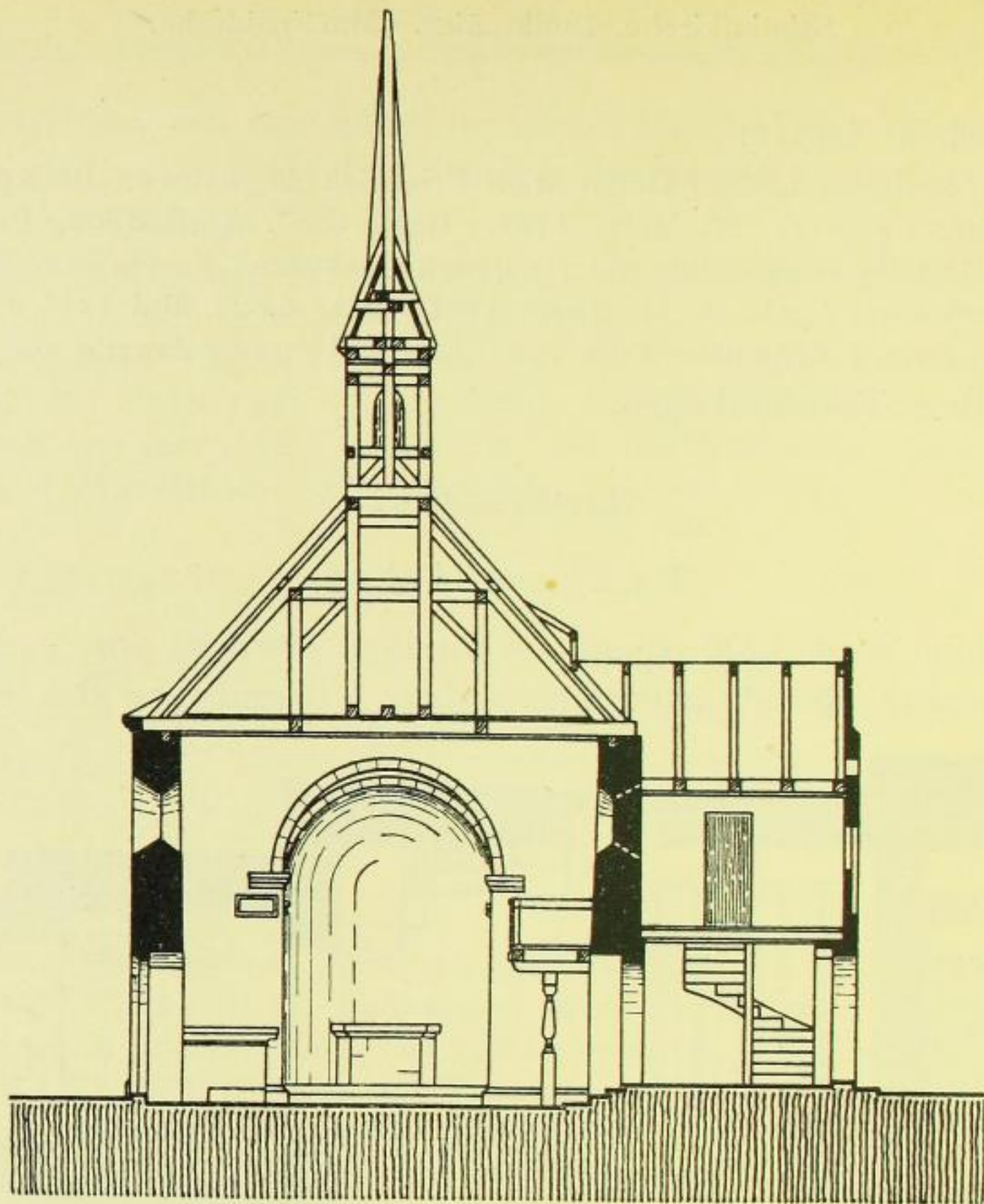
Fig. 193. Martinskirche, Querschnitt
