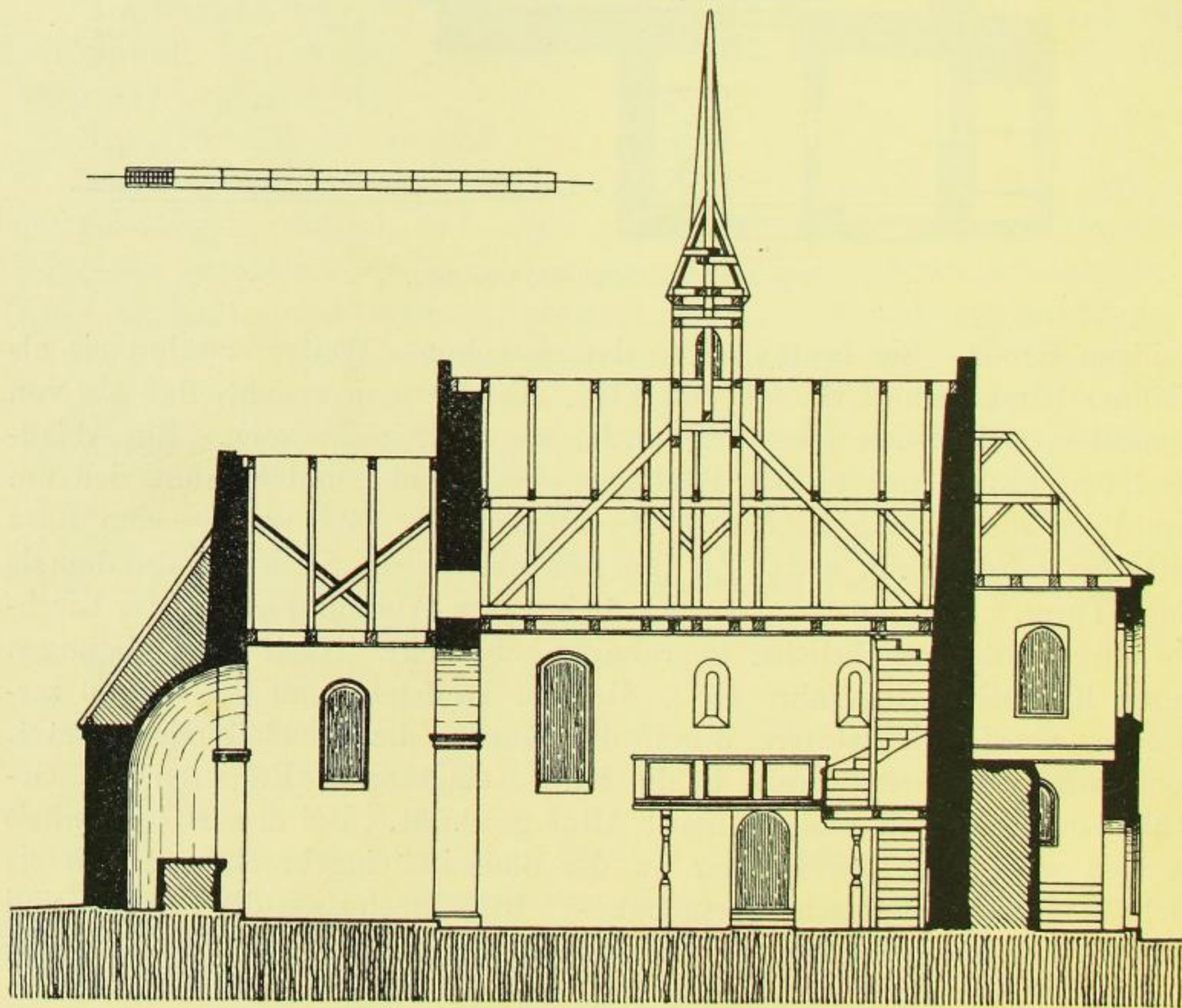
Fig. 194. Martinskirche, Längsschnitt.
