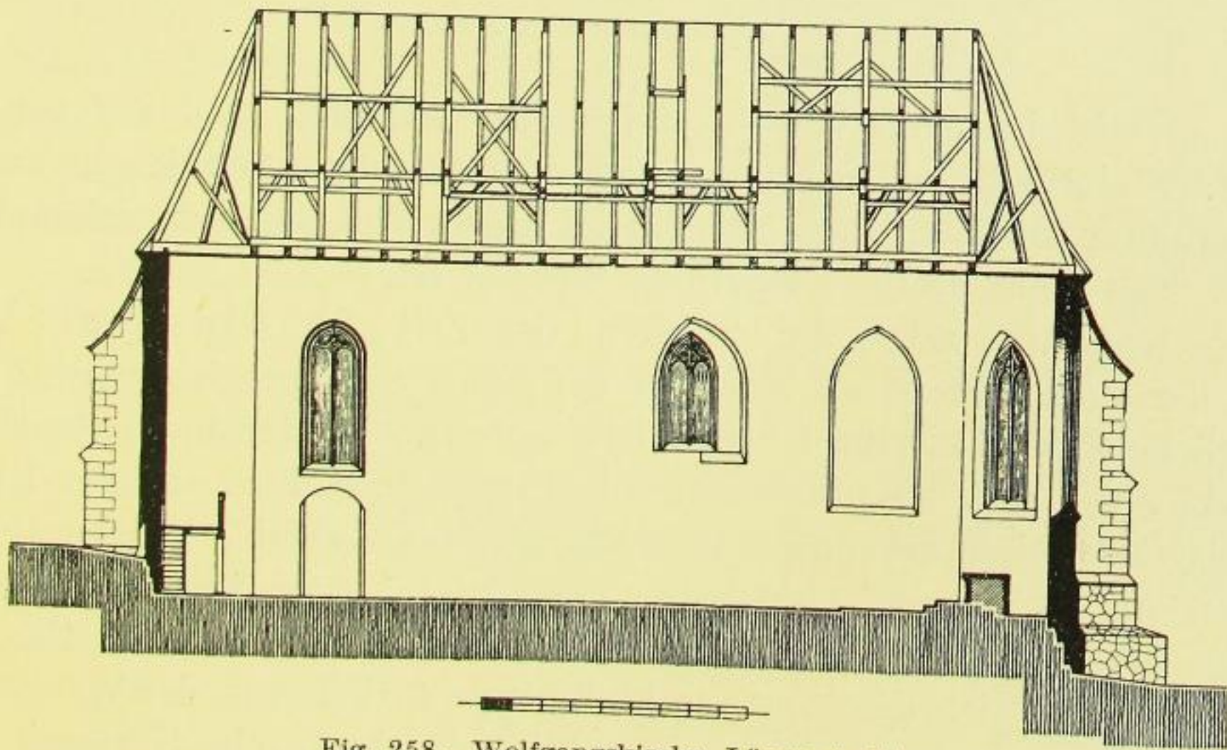
Fig. 258. Wolfgangskirche, Längsschnitt.
