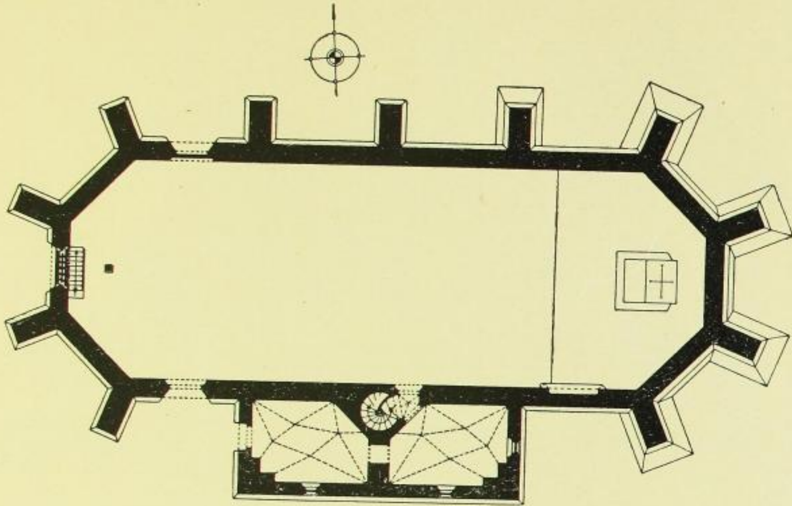
Fig. 256. Wolfgangskirche, Grundriß.
