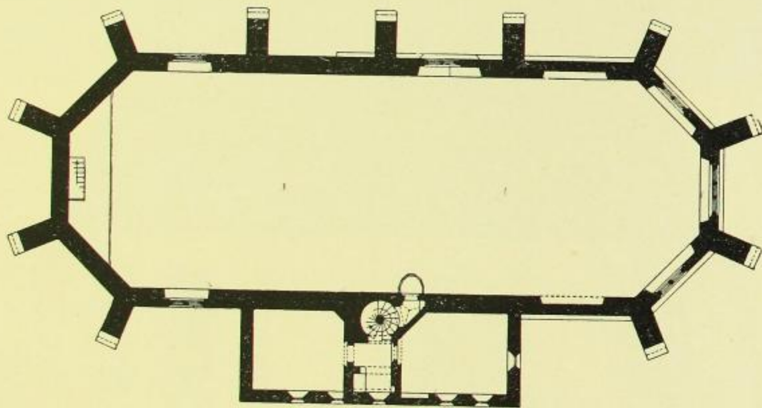
Fig. 257. Wolfgangskirche, Grundriß in Höhe der Empore.
