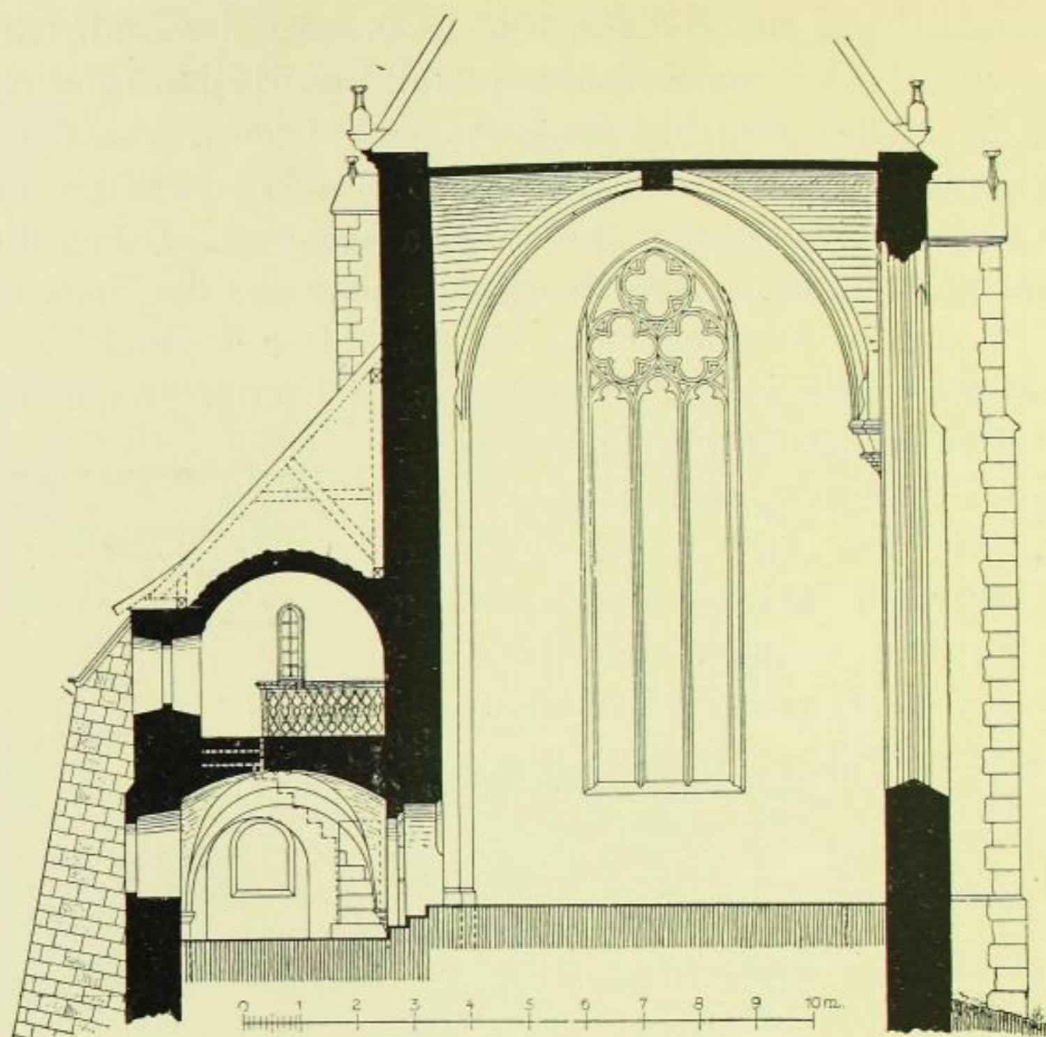
Fig. 515. St. Afra, Querschnitt durch den Chor, die Sakristei und Bücherei.
