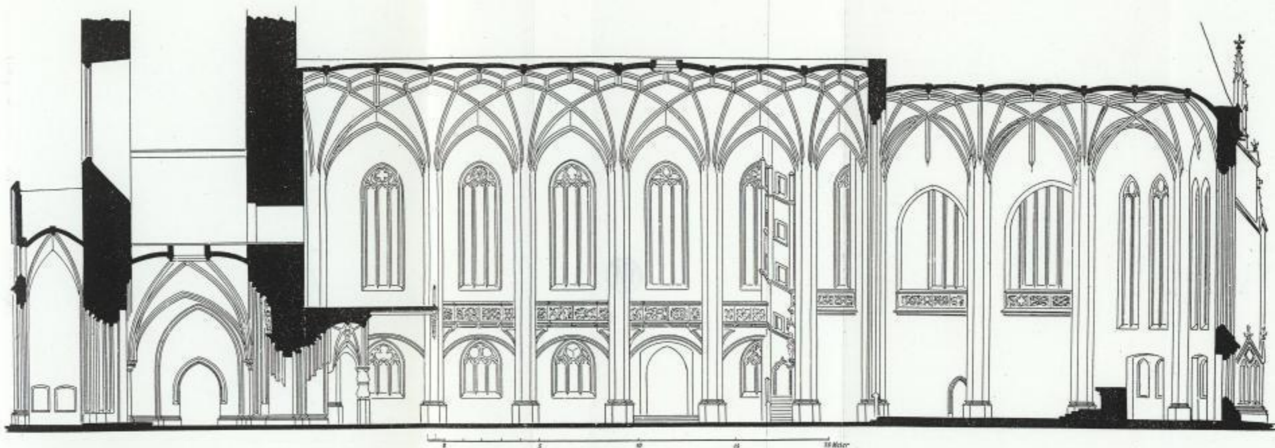
Marienkirche: Längenschnitt.
