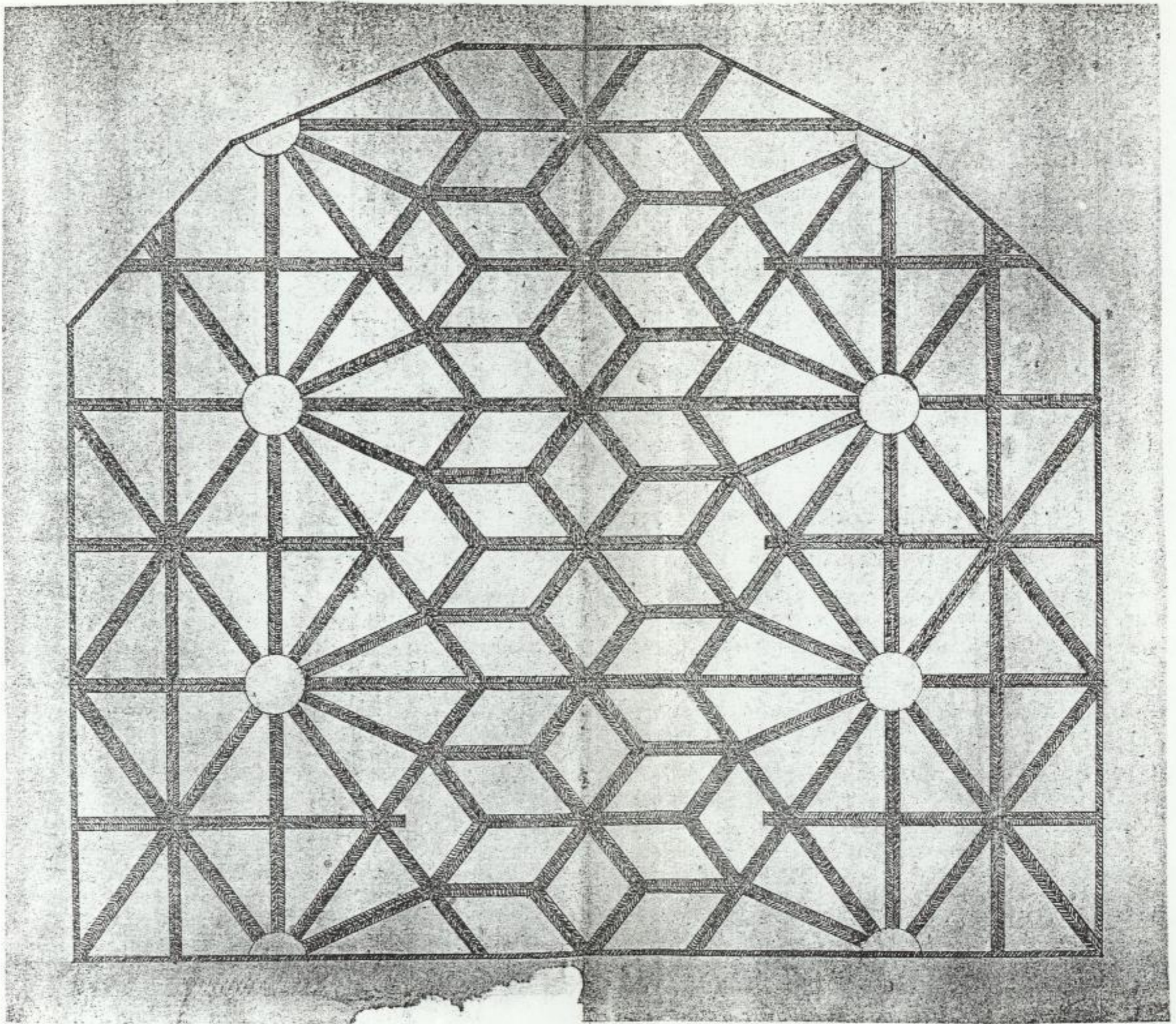
Marienkirche: Facsimile des Gewölbeplans.
