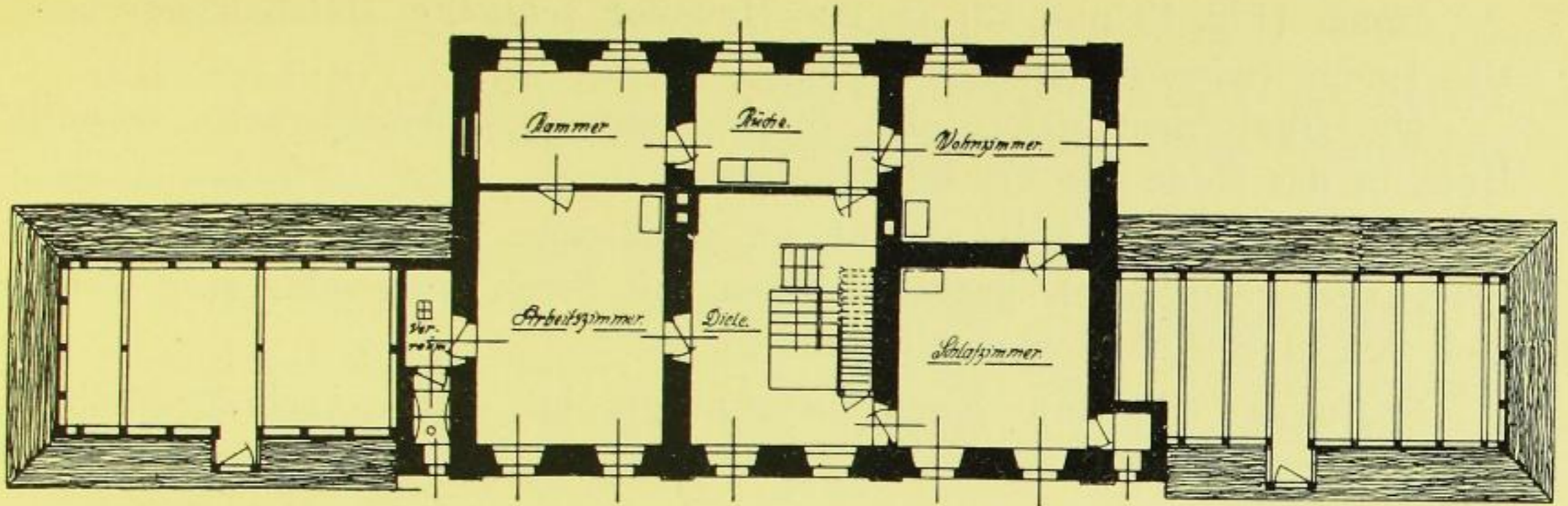
Fig. 12. Bärnsdorf, Teichhaus, Obergeschoß.
