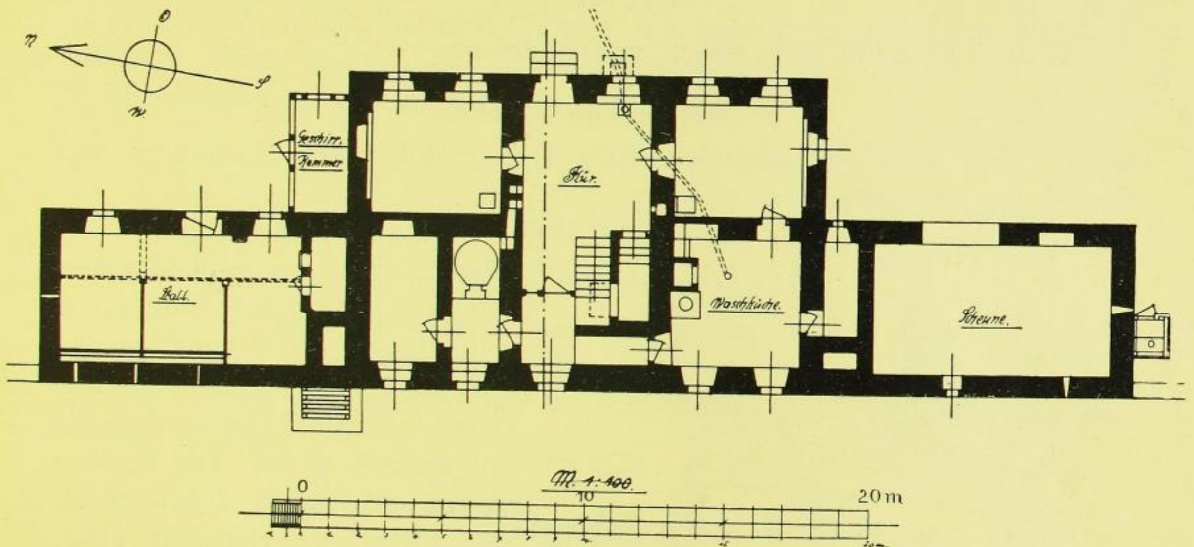
Fig. 13. Bärnsdorf, Teichhaus, Erdgeschoß.
