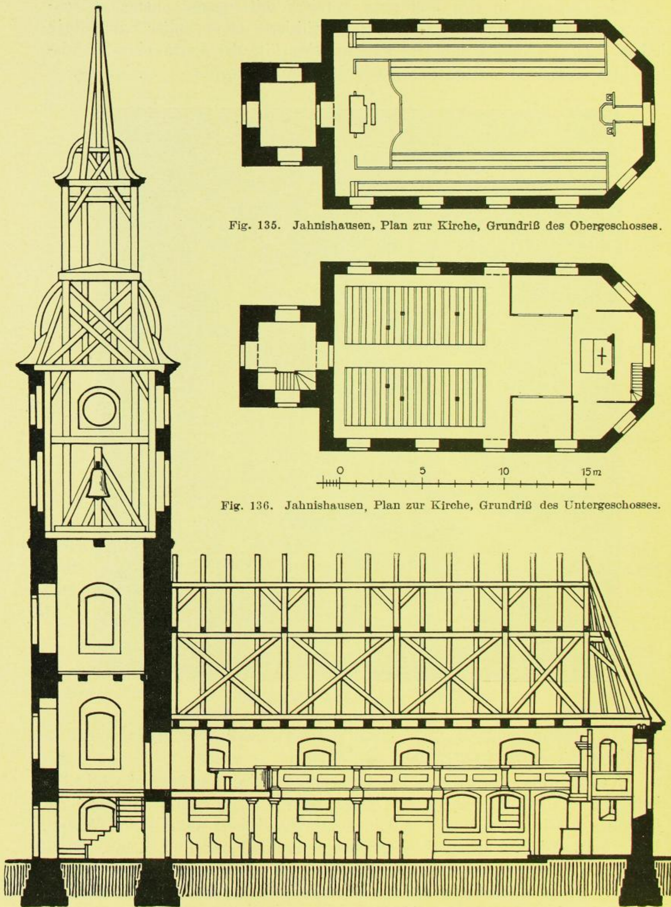
Fig. 137. Jahnishausen, Plan zur Kirche, Längsschnitt.
