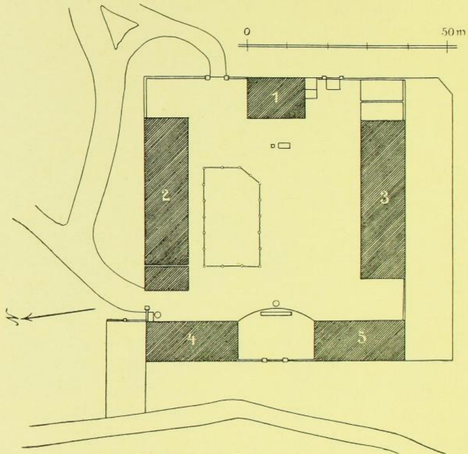
Fig. 154. Kalkreuth, Reierhof, Lageplan.
