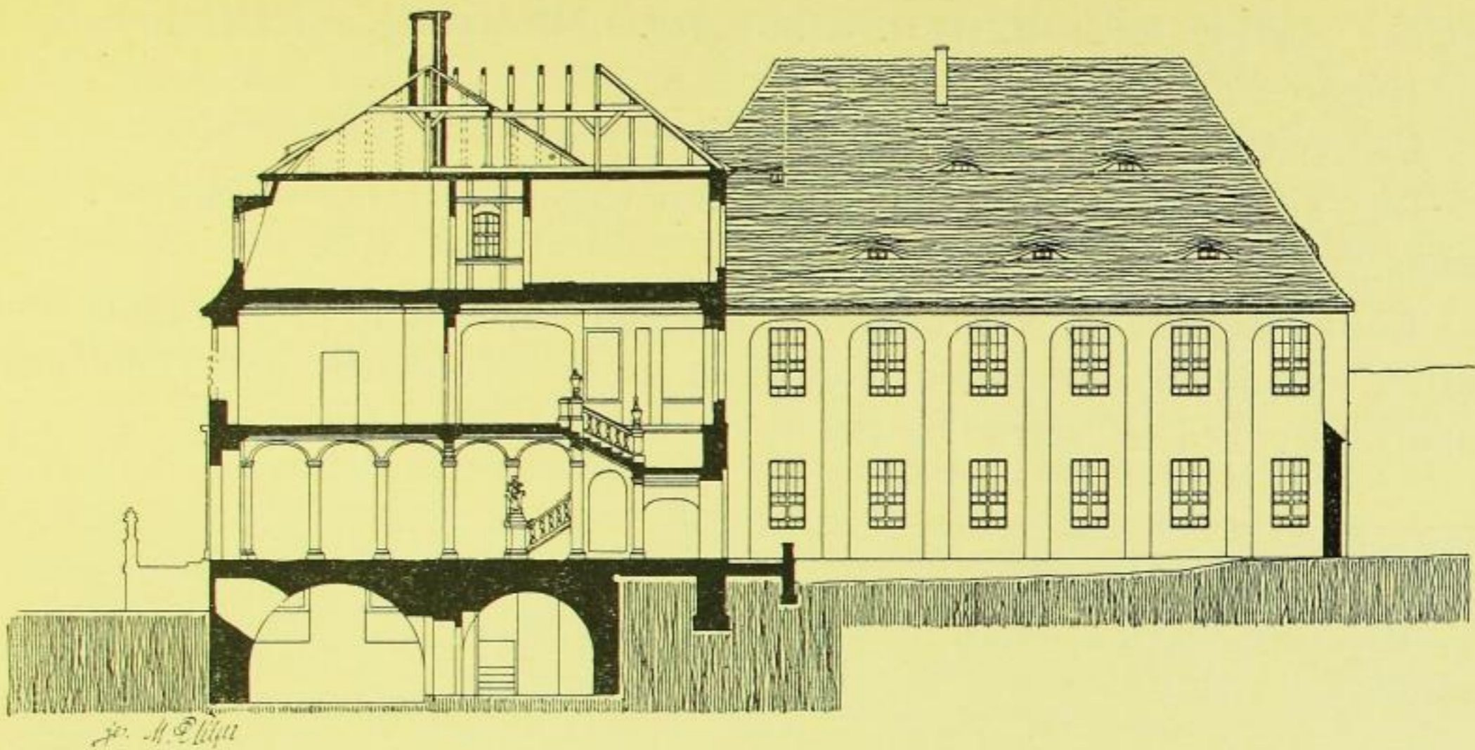
Fig. 402. Seußnitz, Schloß, Querschnitt.
