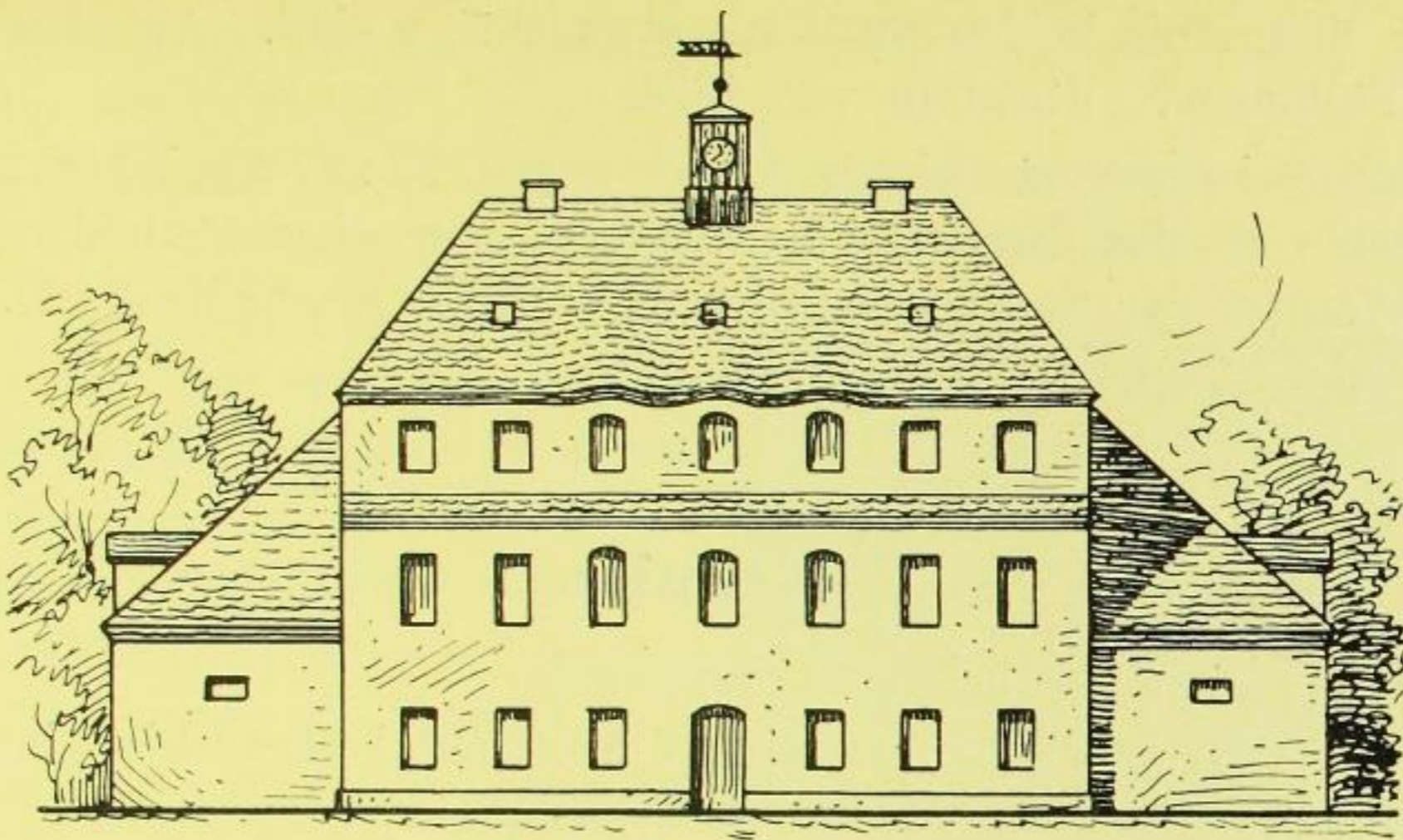
Fig. 521. Weißig, Forsthaus, Vorderansicht.
