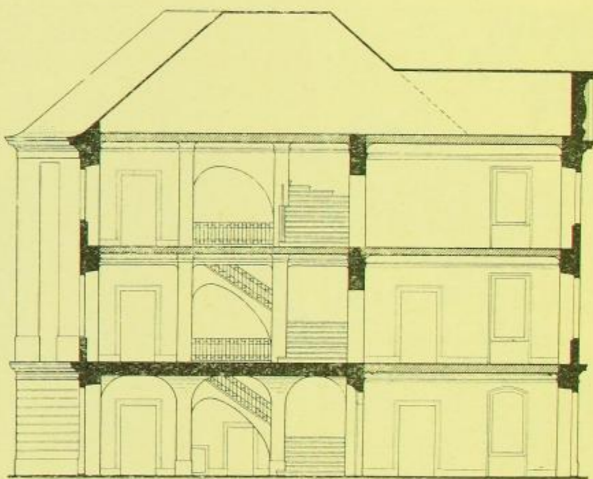
Fig. 557. Zabeltitz, Palais, Schnitt.
