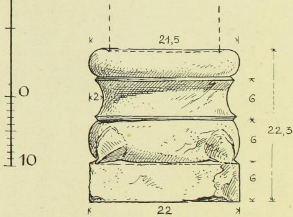
Fig. 12. Kämpferstein. Fig. 13. Säulenfuß.
