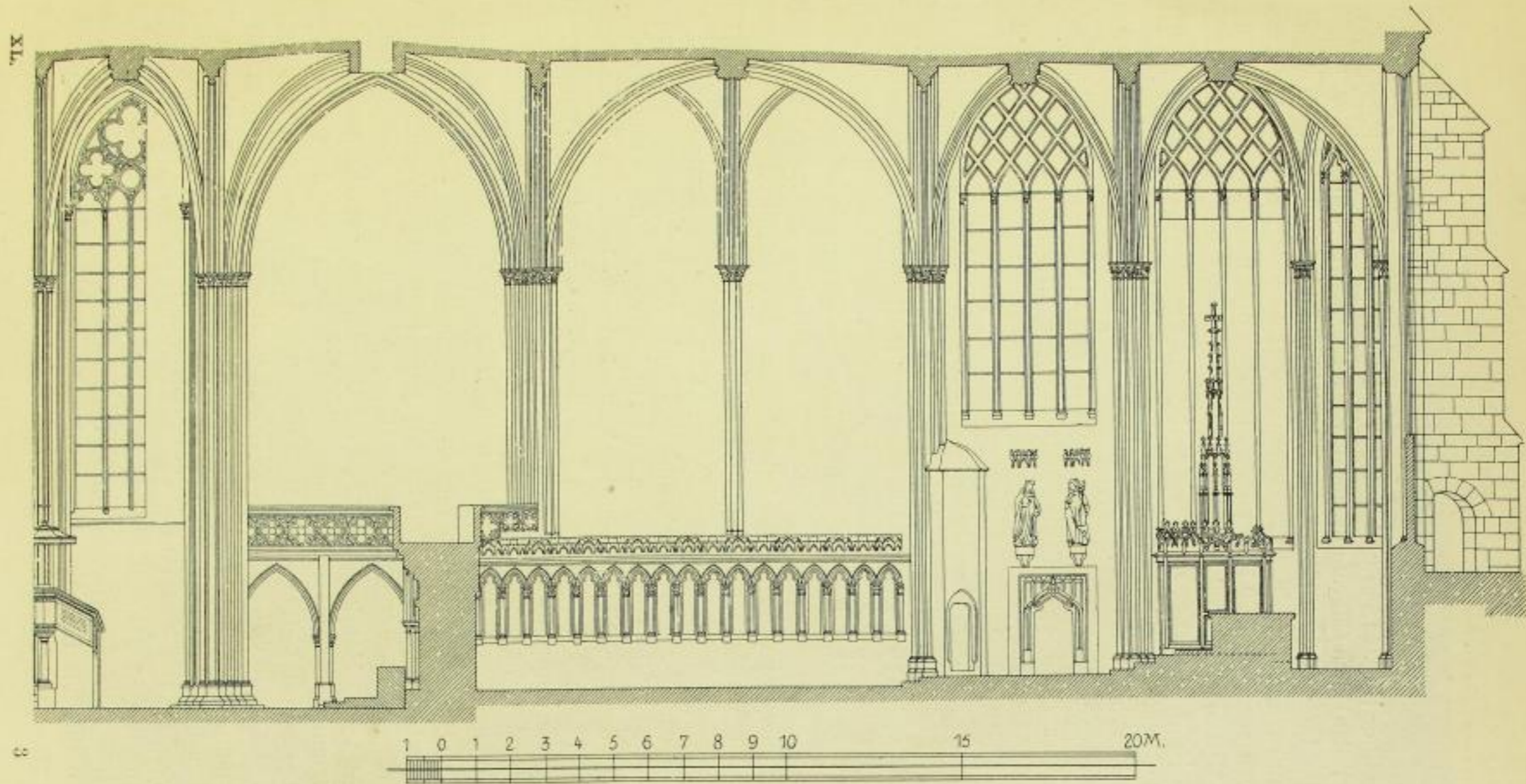
Fig. 44. Meißner Dom, Schnitt durch das Querhaus und den Chor.
