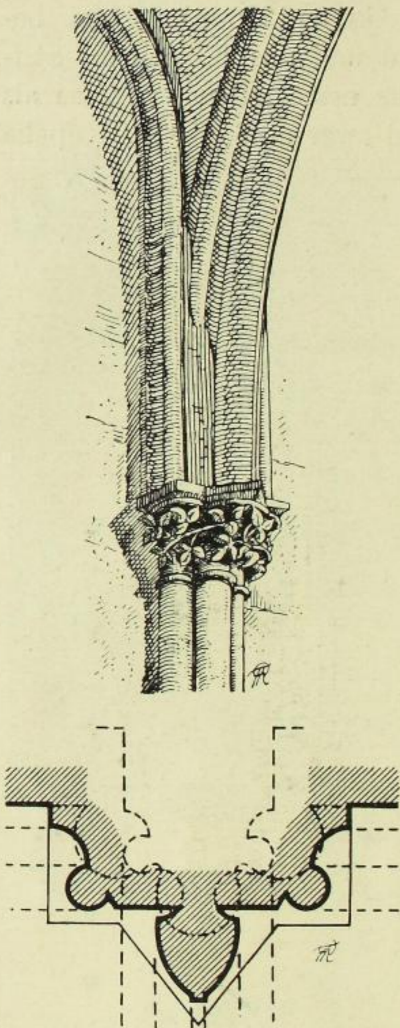
Fig. 62 und 63. Gewölbeanfänger des sechsteiligen Gewölbes mit dem Kämpfer-Grundriß. Nördliche Zwischenrippe.
