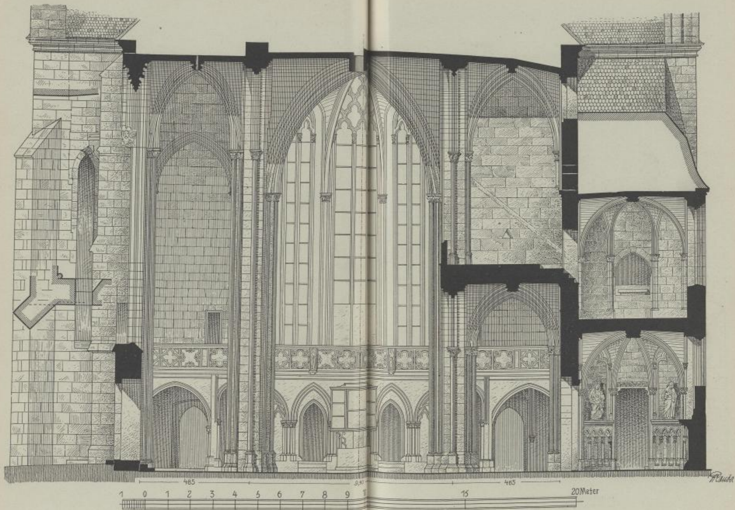
Querschnitt durch das erste Langhausjoch und den Achteckbau.
