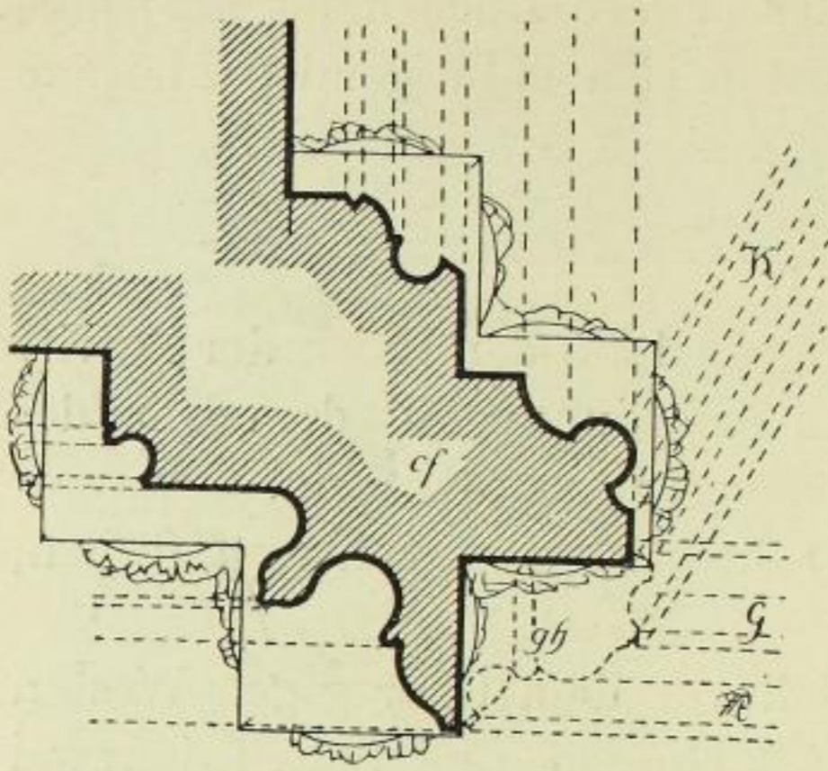
Fig. 95. Kämpfergrundriß, Linie c—f in Fig. 96.
