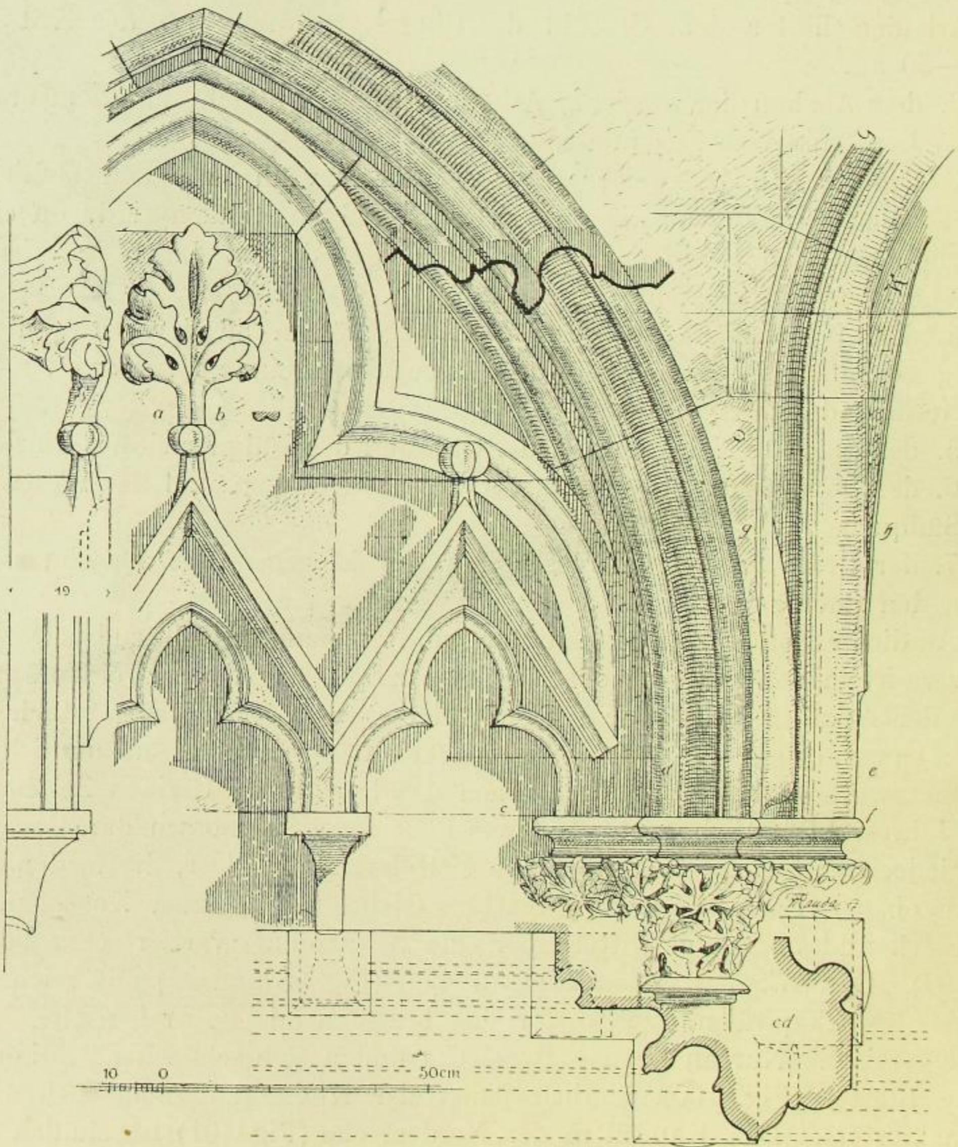
Fig. 96. Südwestecke am Mittelteil des Lettners.
