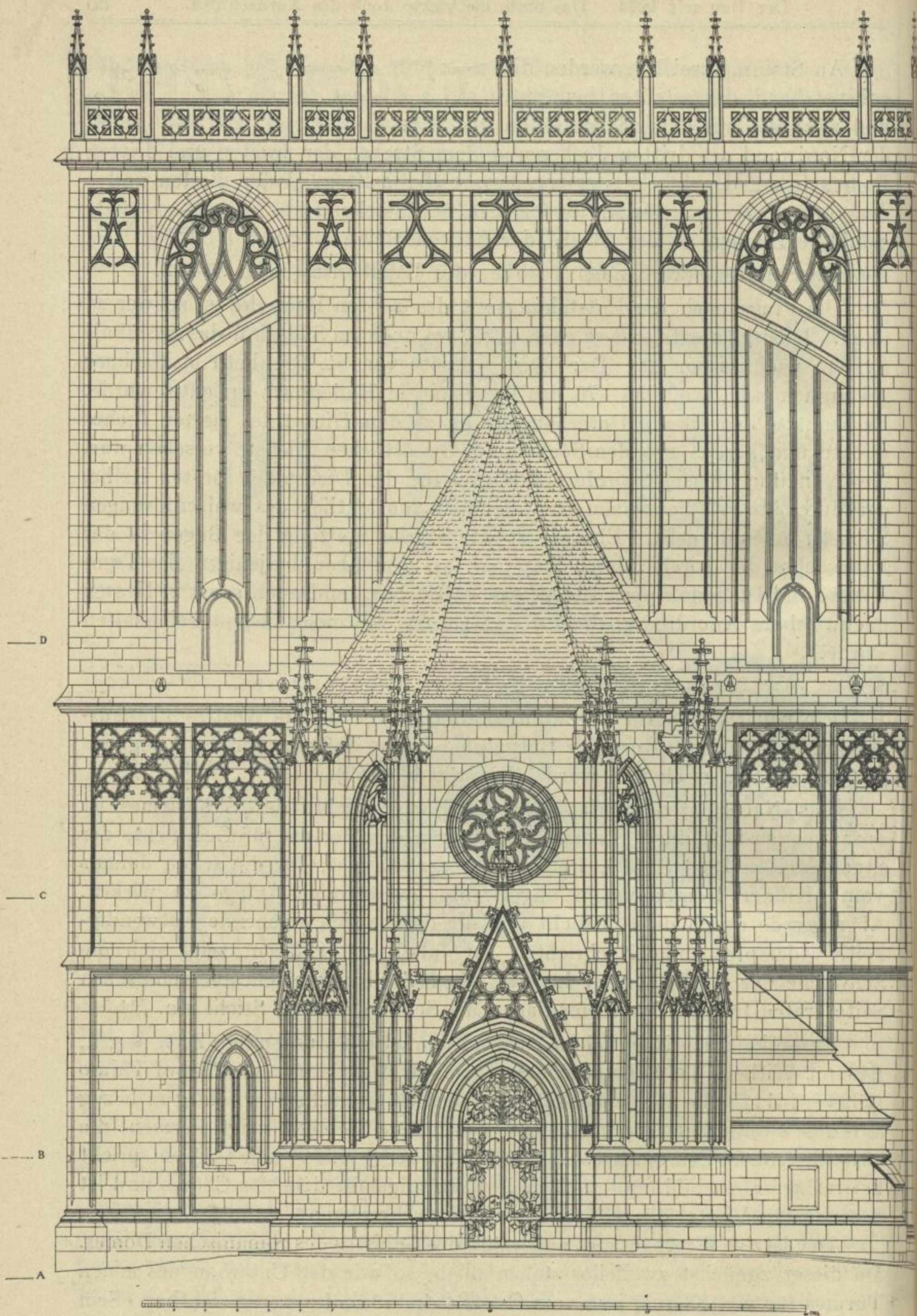
Fig. 139. Westansicht des Domes, Fürstenkapelle und Westturm (Meßbildaufnahme).
