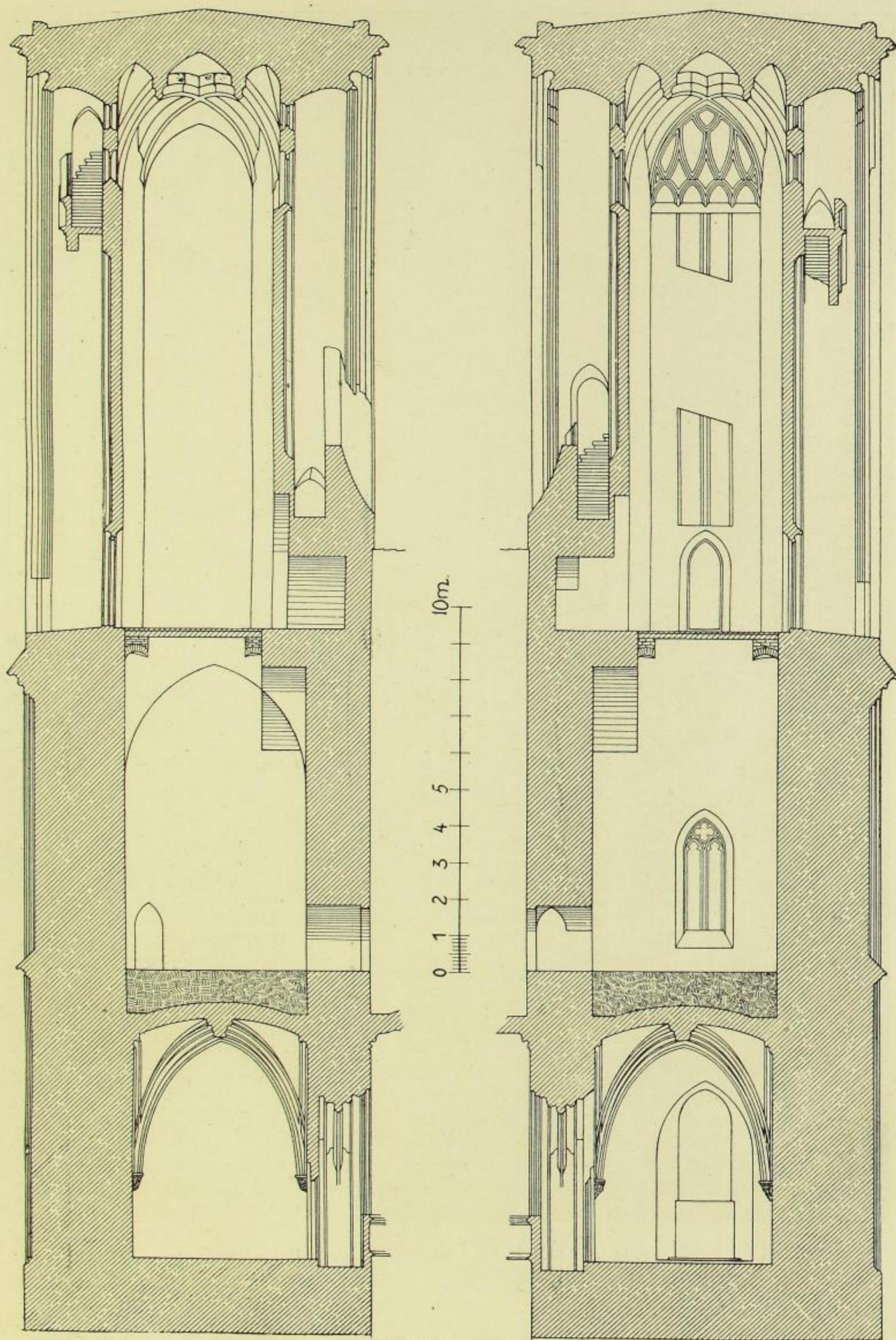
Fig. 187. Schnitt durch den Südteil des Westturmes, Blick nach Norden.
